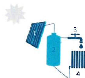
1 Zonnecollector | 2 Opslagvat zonnecollector 3 Sanitair warm water 4 Warmte afgeven naar ruimteverwarming
