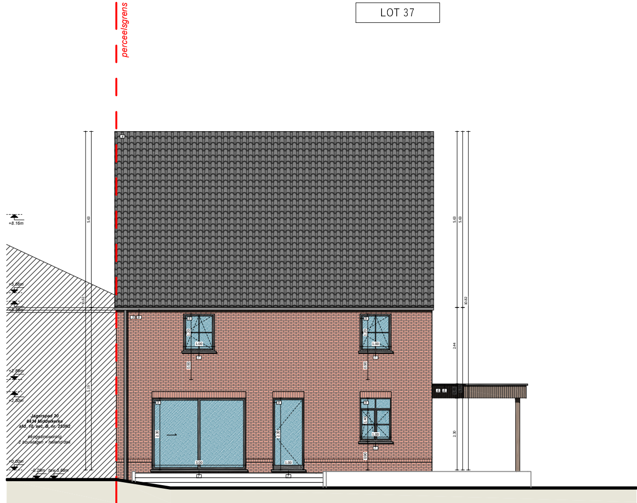
lot 35B, 36, 37 & A achtergevel 0 1 2 3 4 5 1:50 1:50
