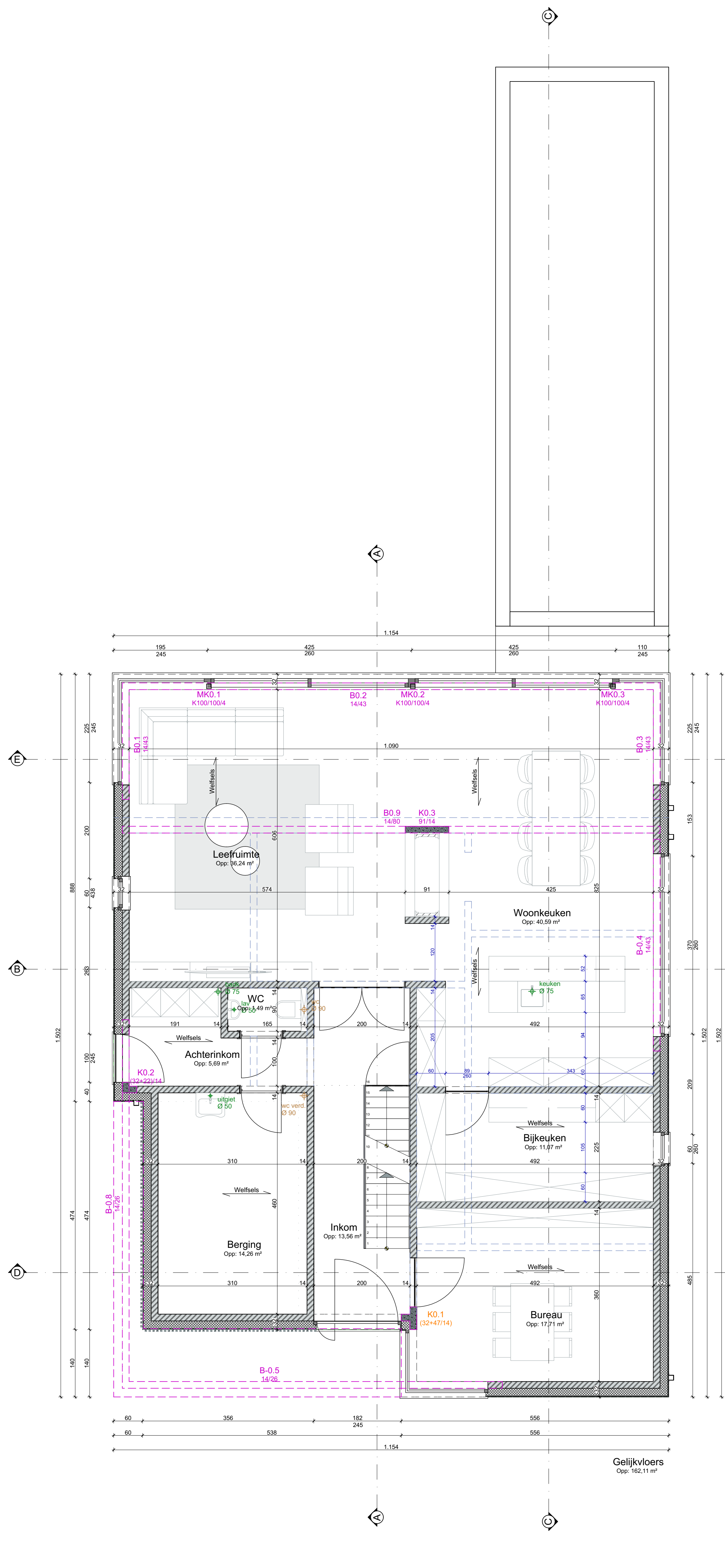
Gelijkvloers 1:50
