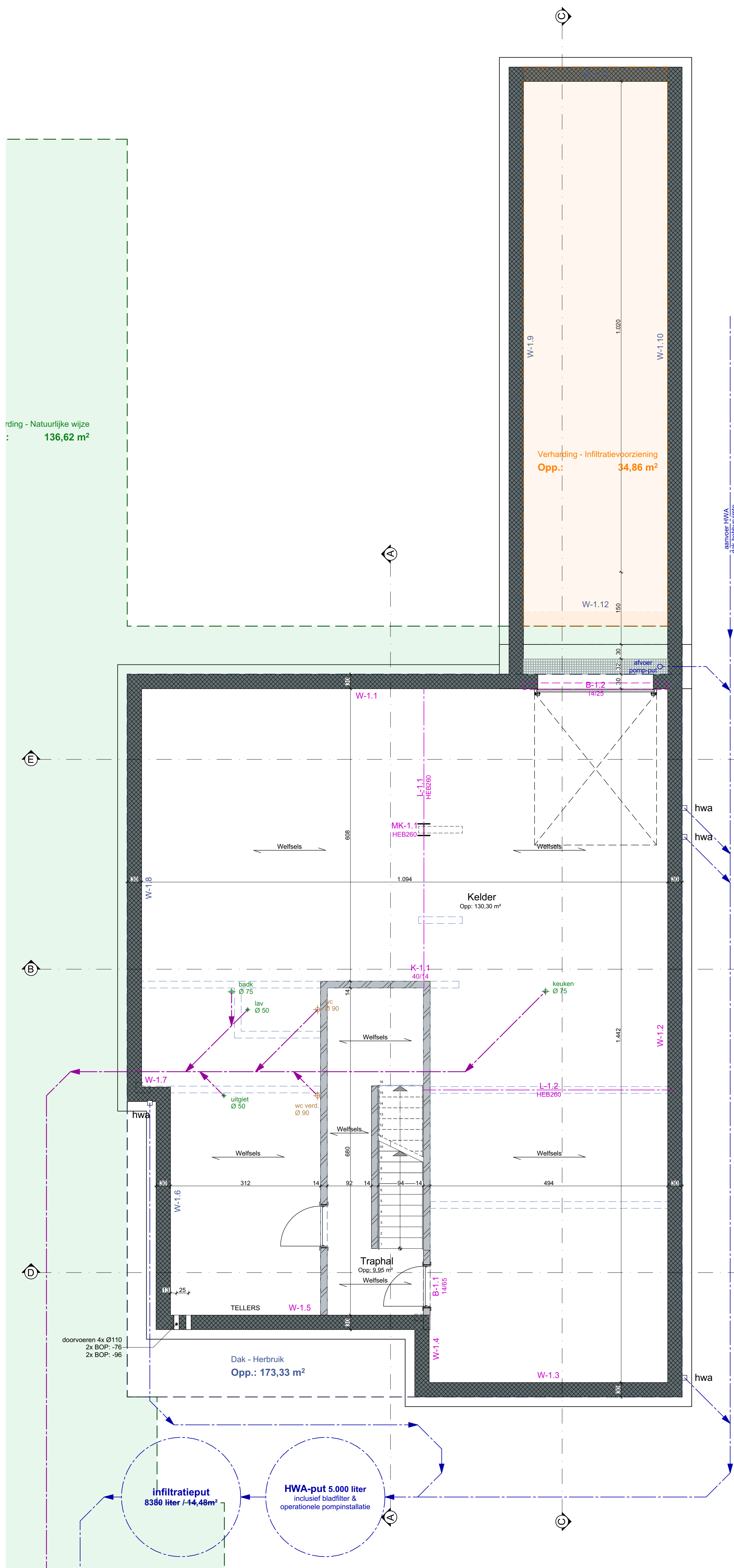
Kelder 1:50
