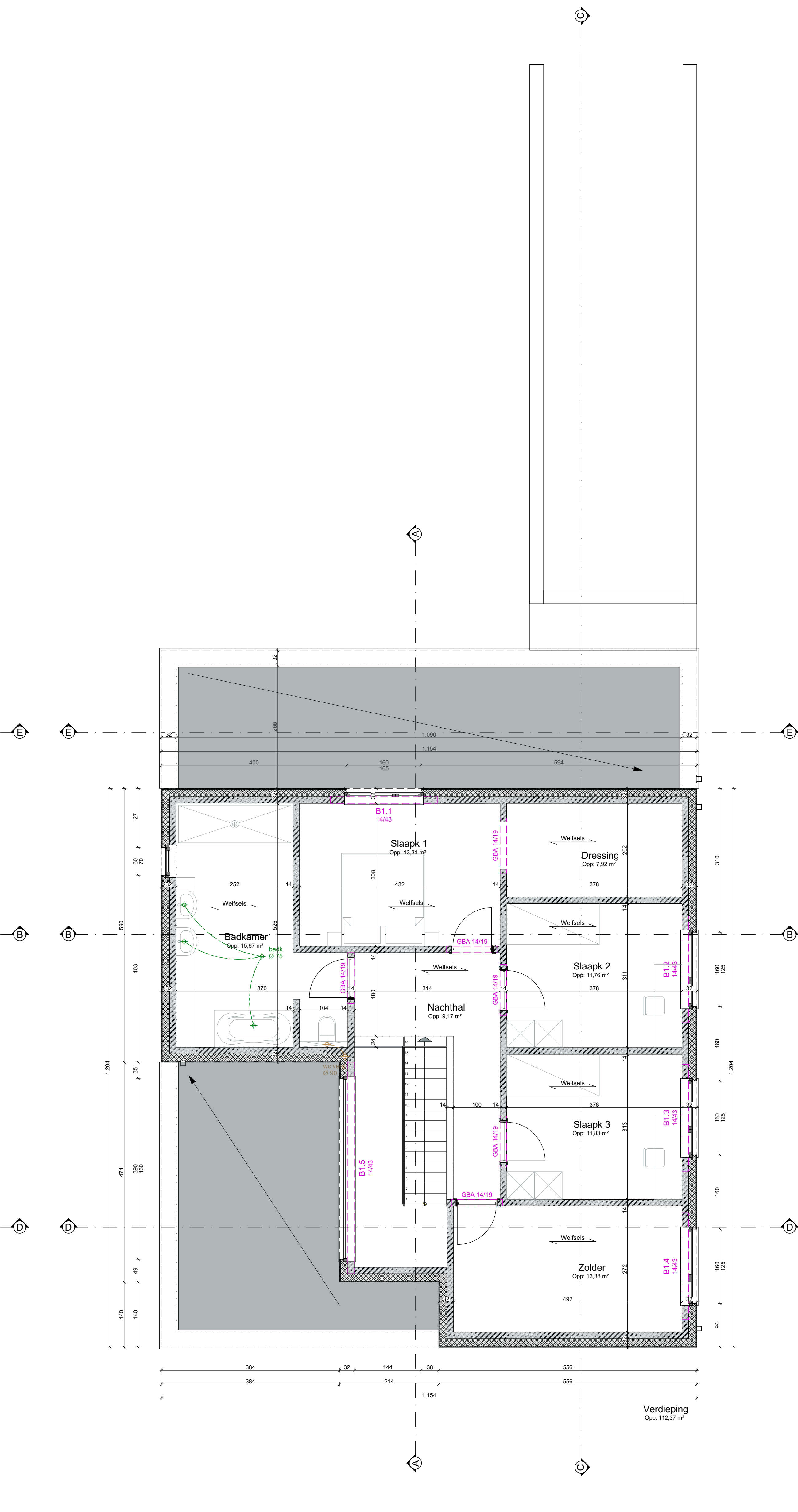
1e verdieping 1:50
