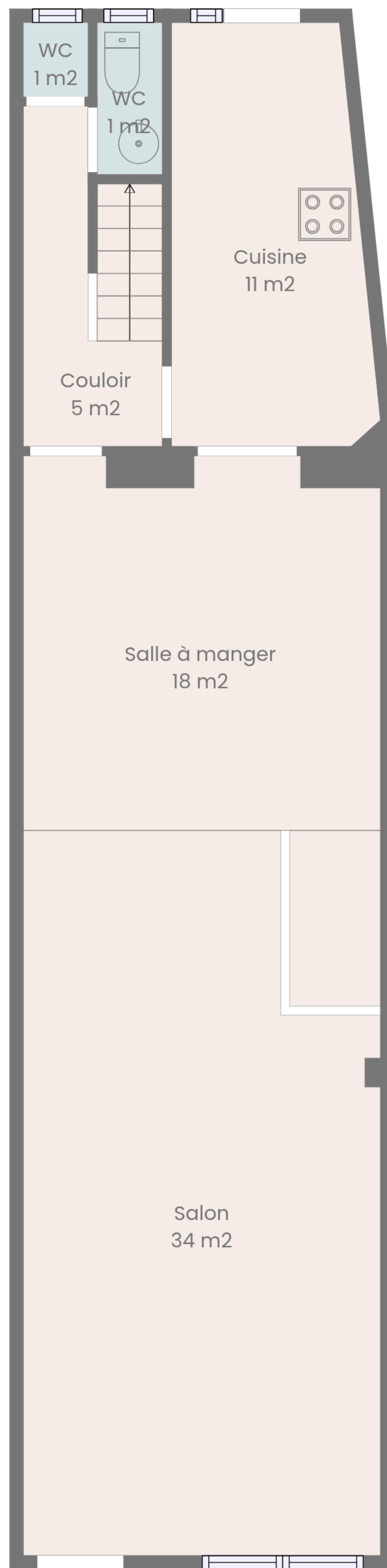
Rez-de-chaussé
