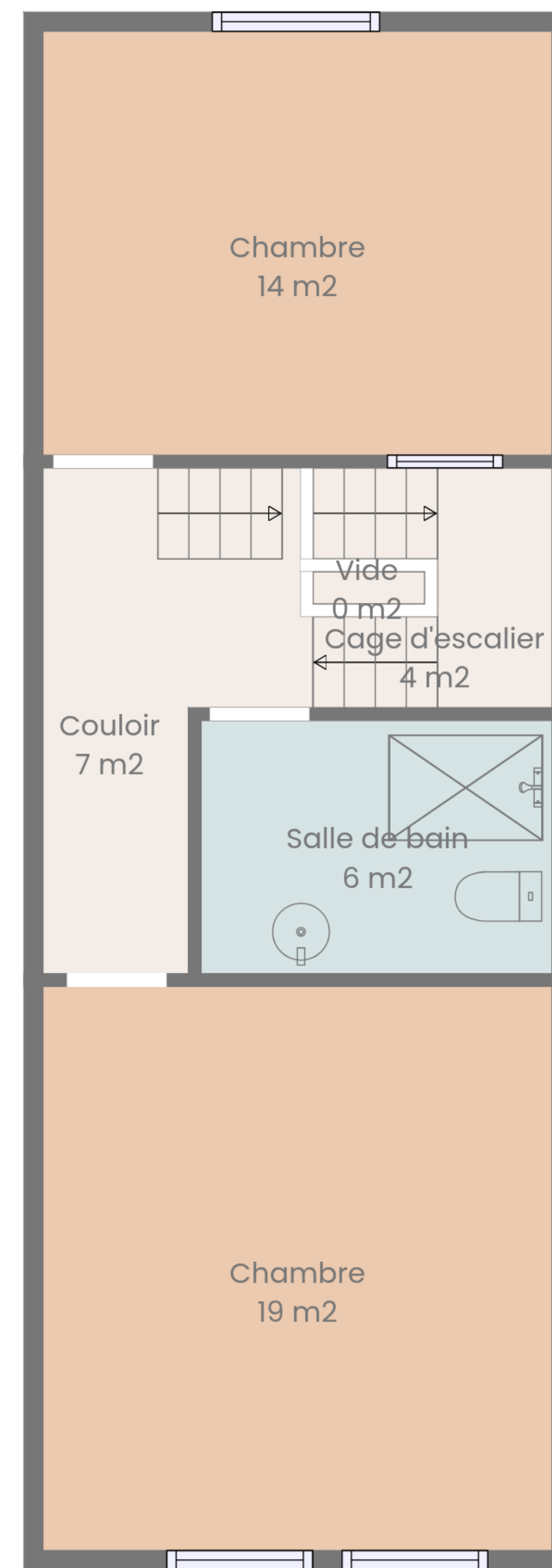
2ème étage
