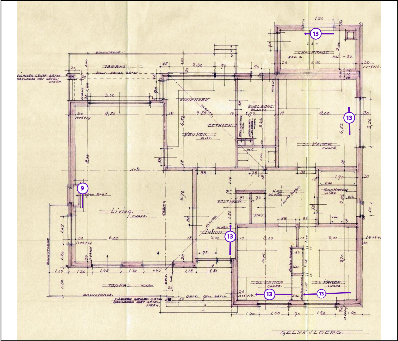
Legende van plan 1.2: Gelijkvloers plaatradiatoren - haardcassette
