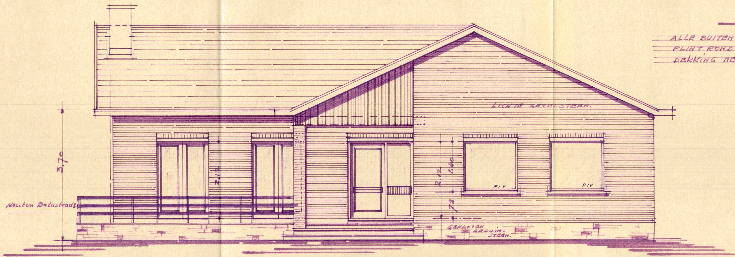
Voorgevel.
