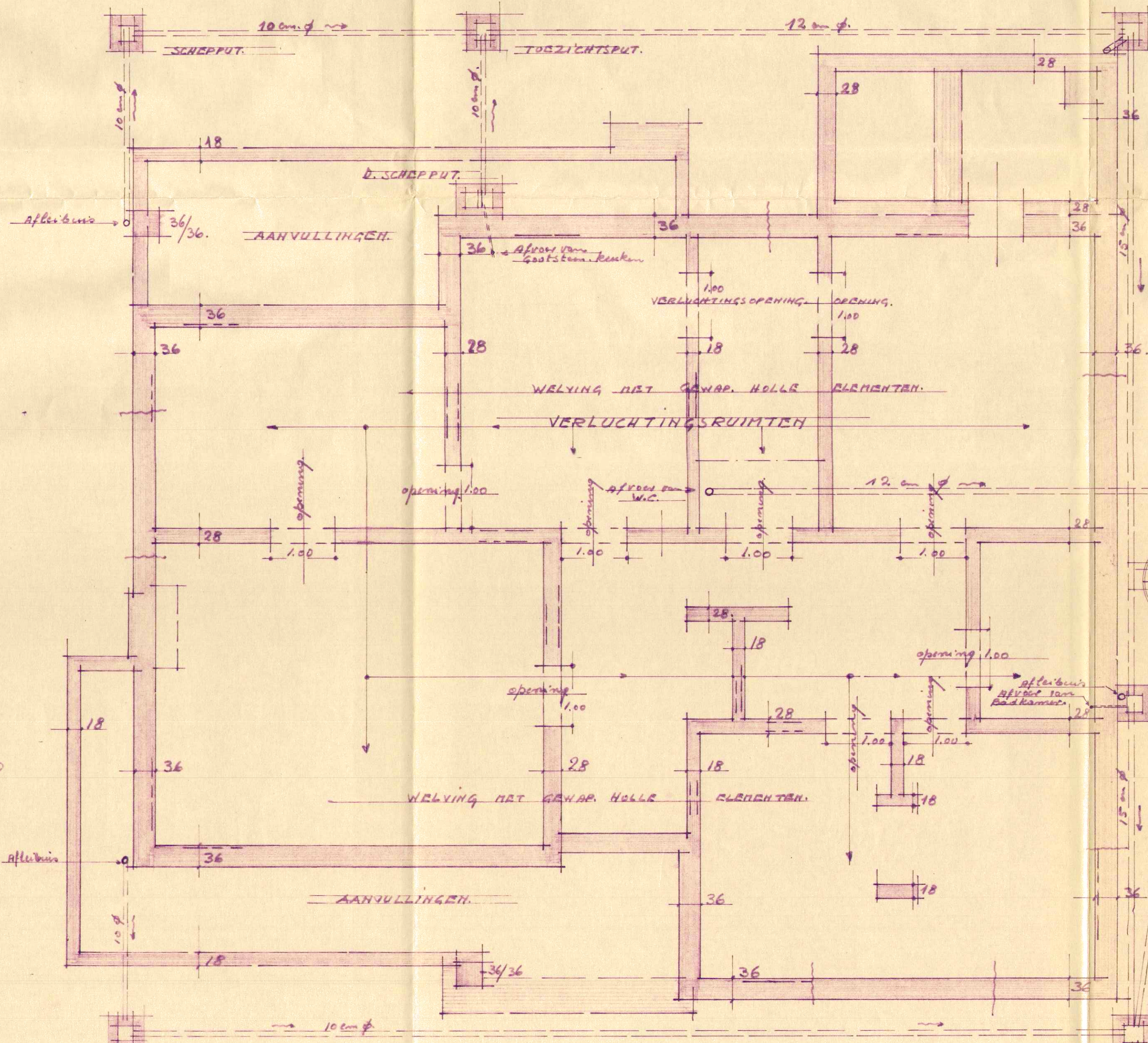
Fonderingen.
