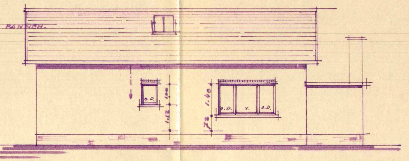
Zygevel, Rechts.
