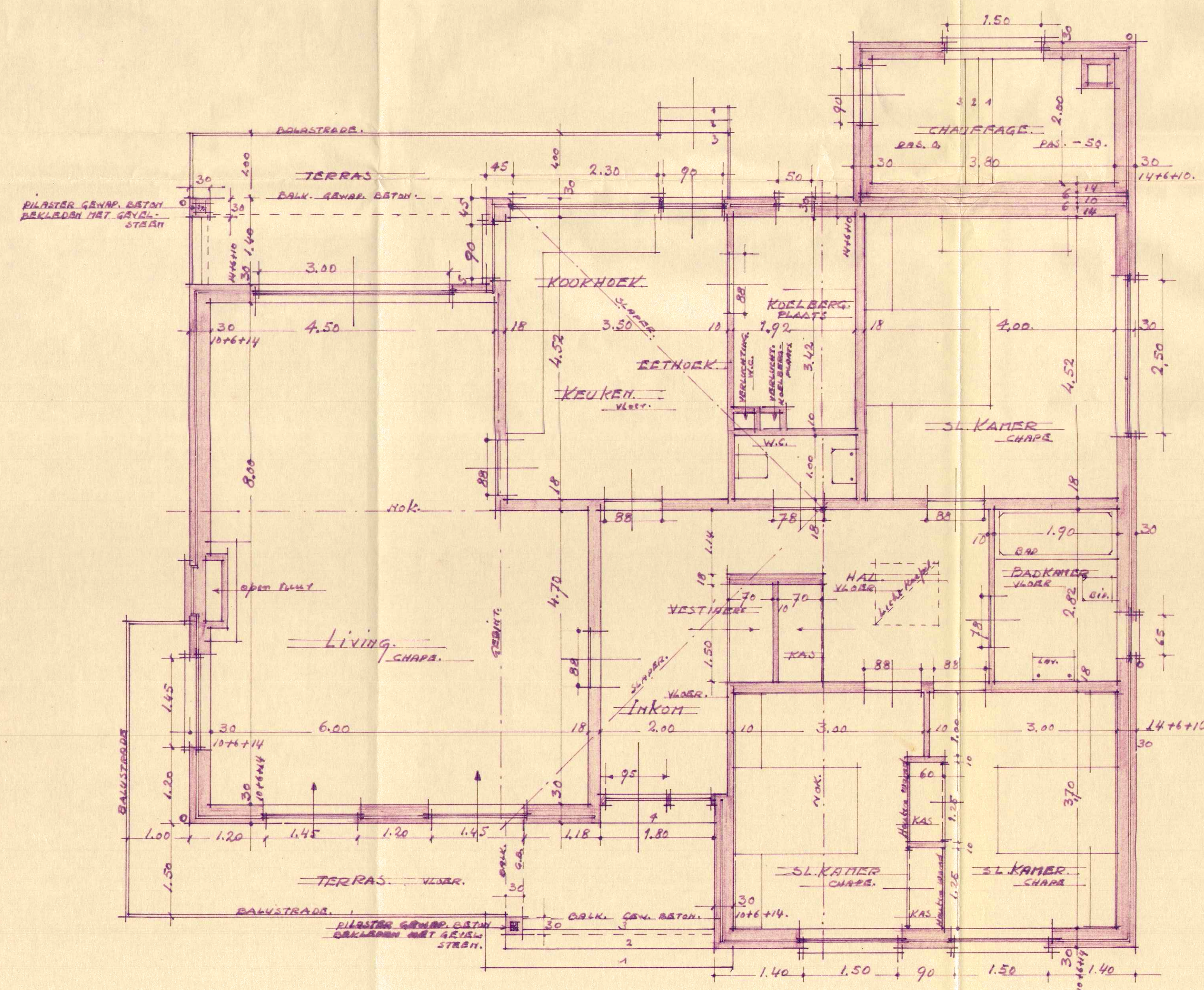
Gelykvloers.
