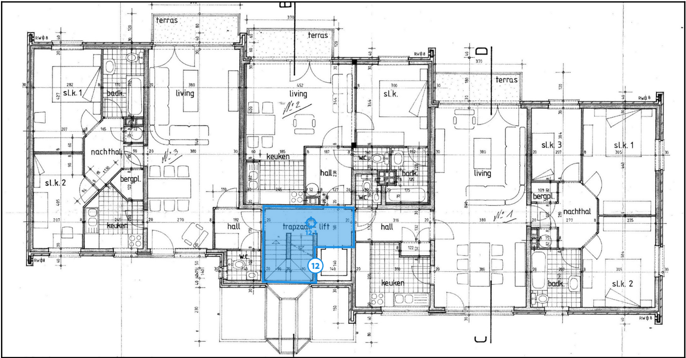
Legende van plan 1.9: Verdieping +5
