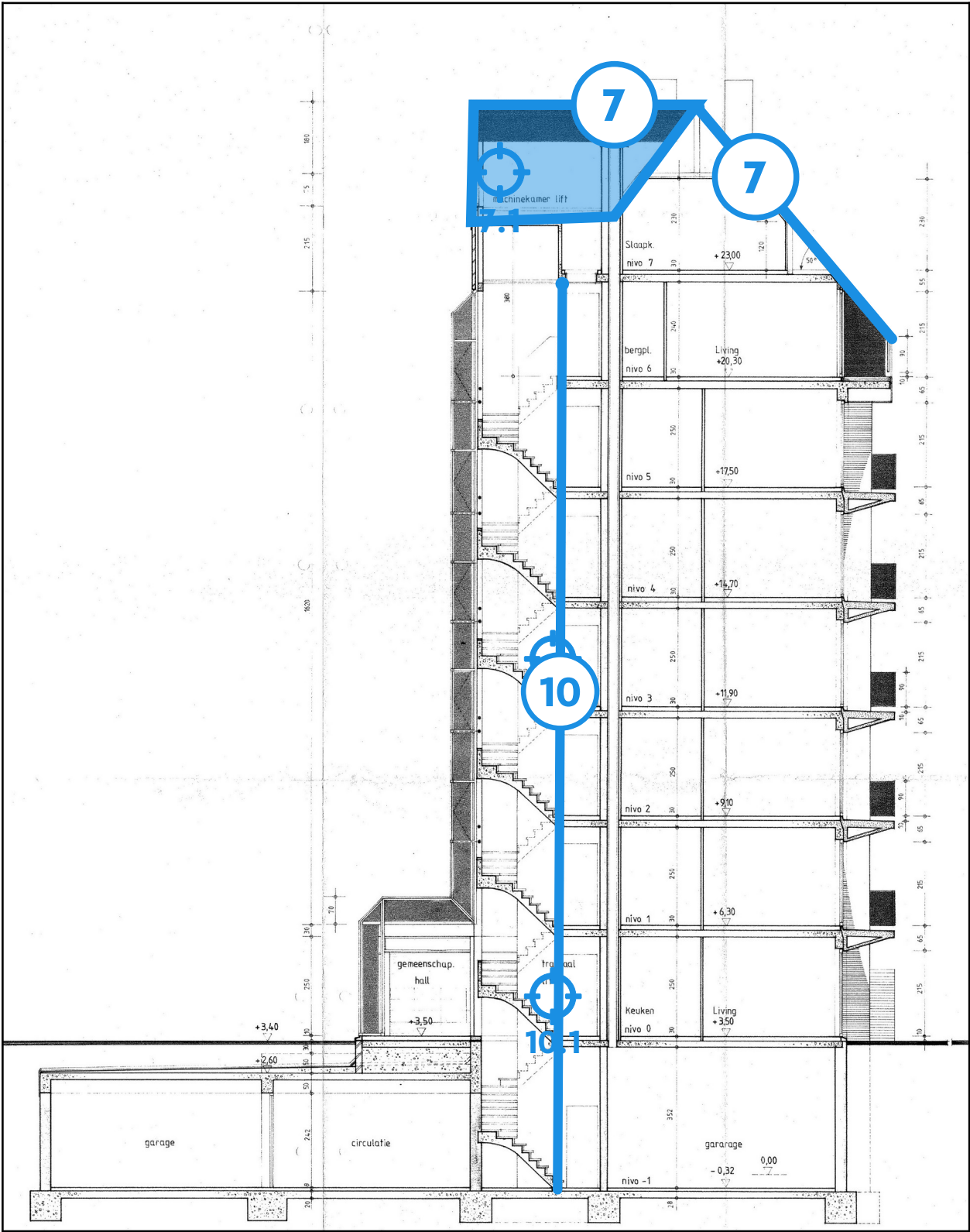
Legende van plan 1.16: Doorsnede
