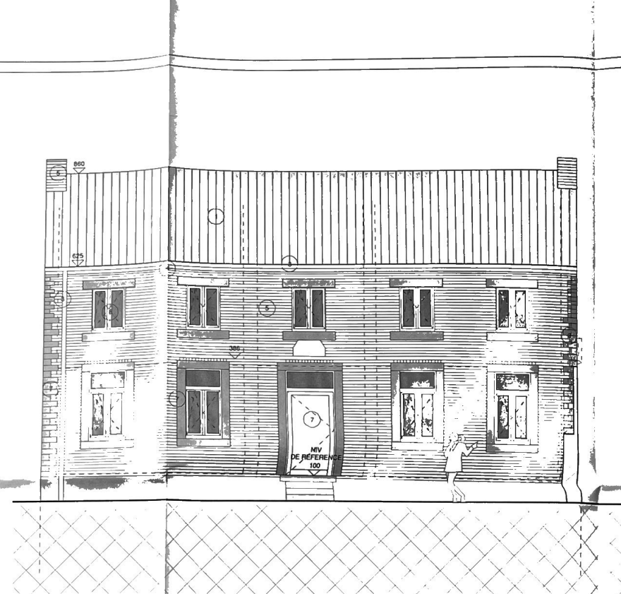
Facade avant
