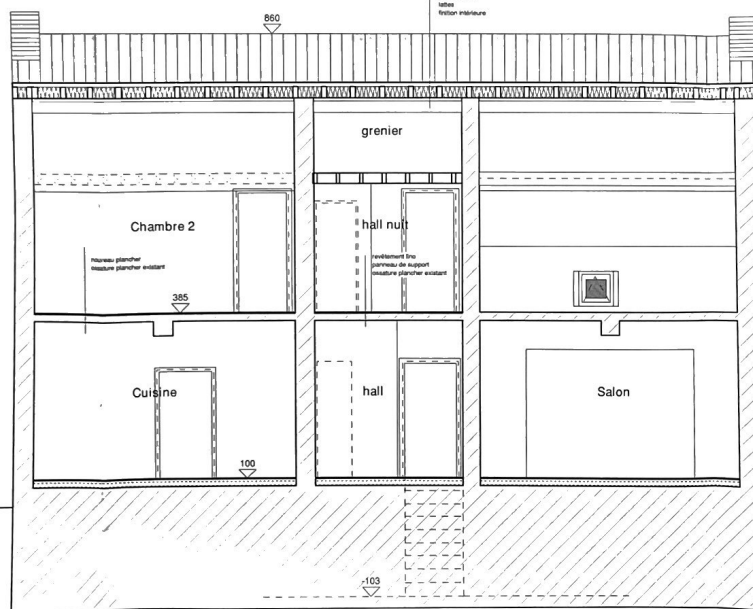
Coupe AA
