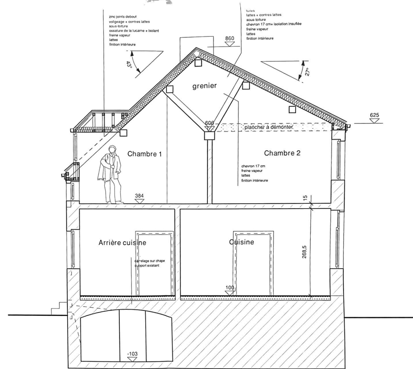
Coupe CC
