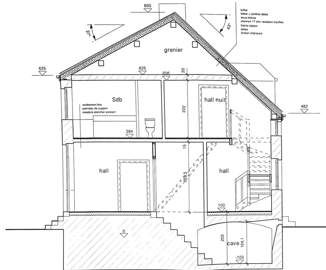
Coupe BB
