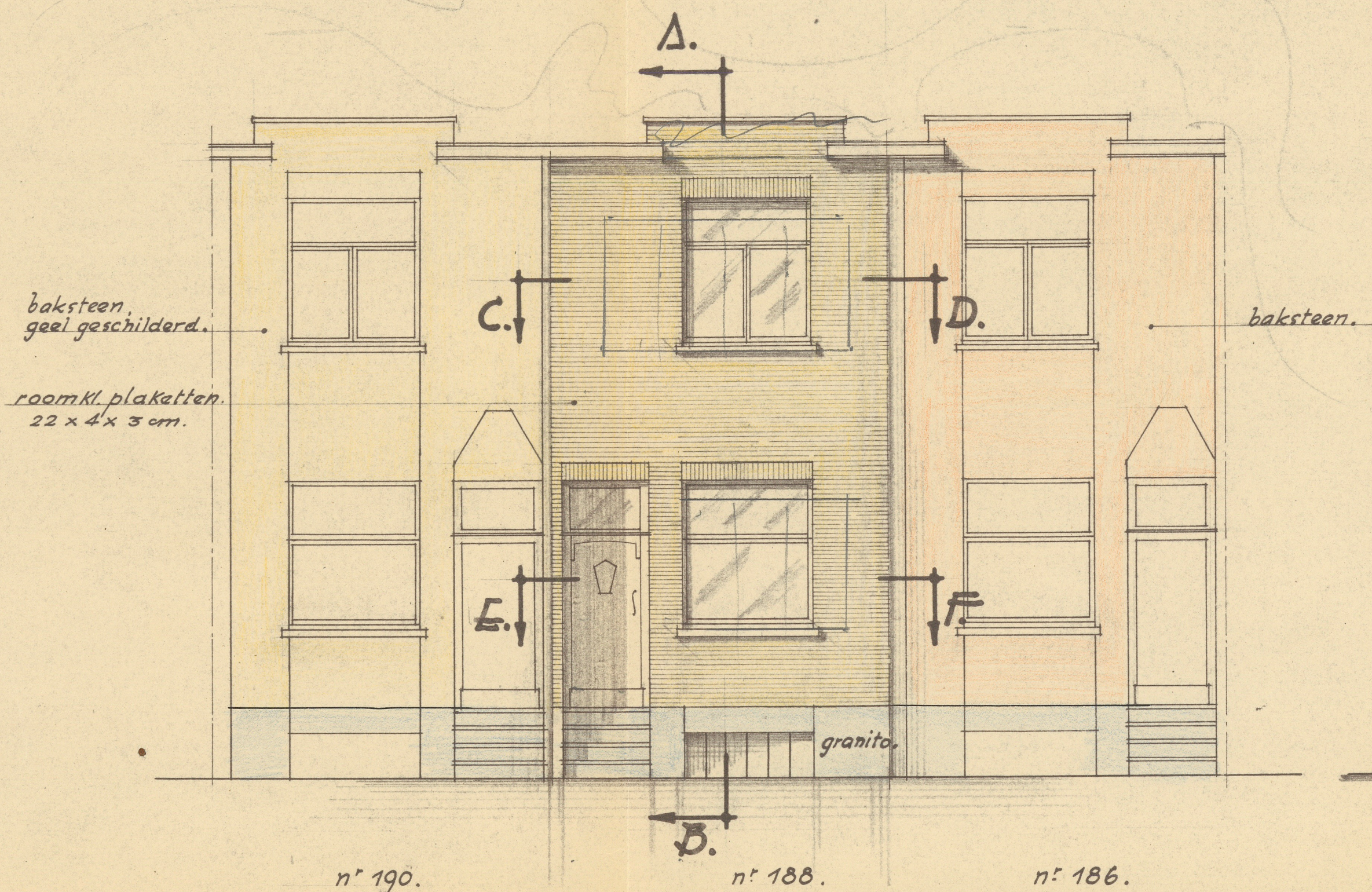
Nieuwe Voorgevel.
