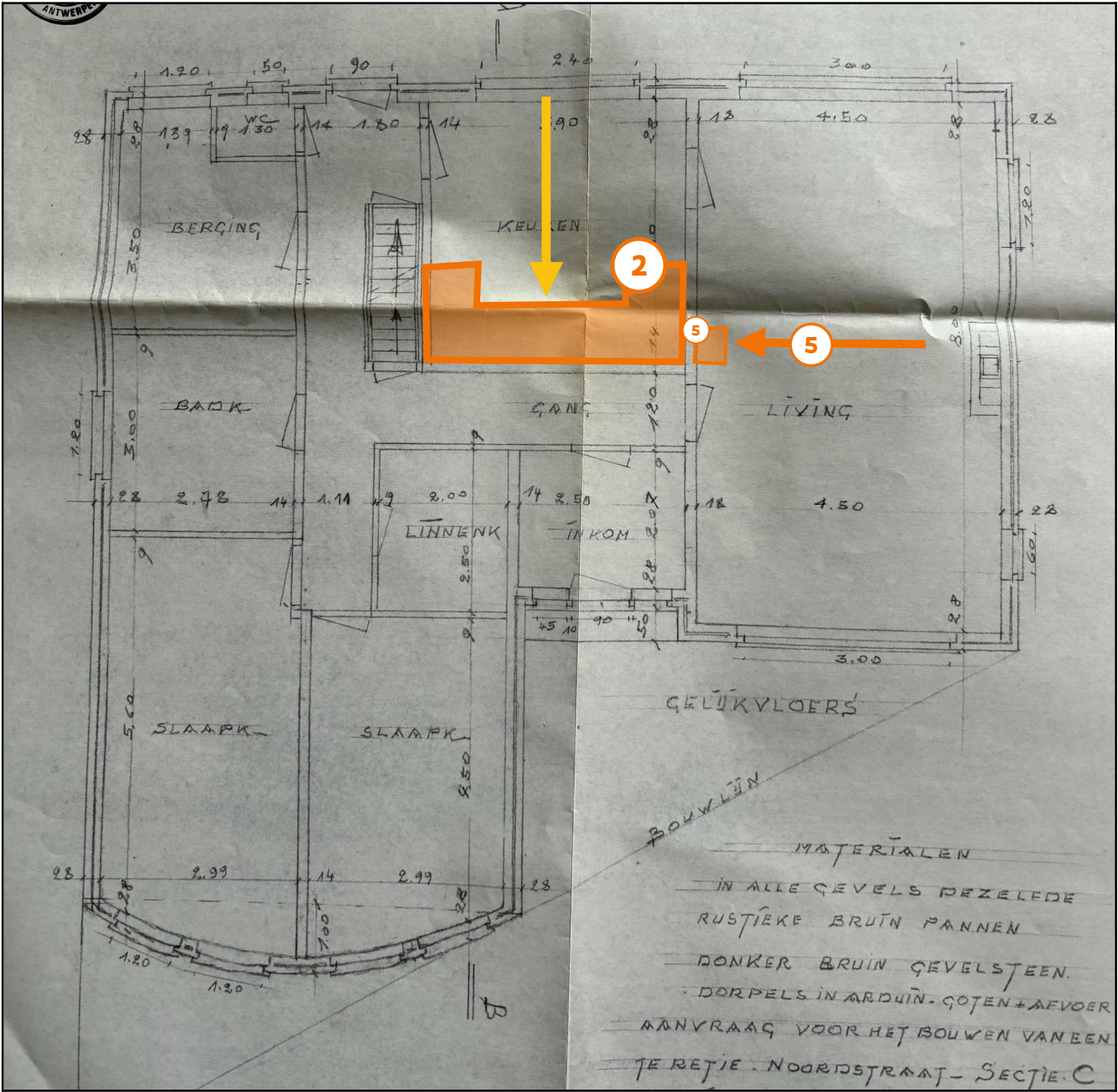
Legende van plan 1.1: akoestische isolatie onder afdruiptak
