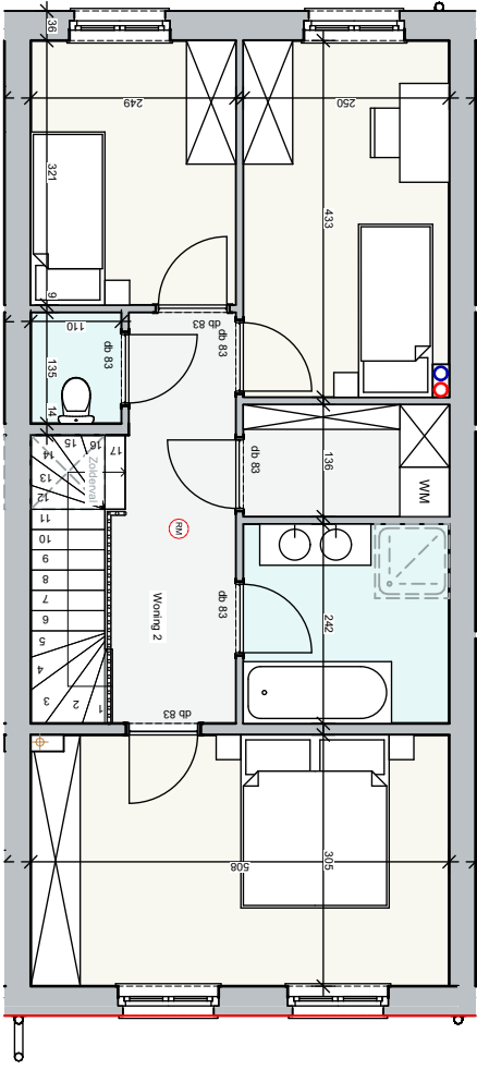
Eerste verdieping
