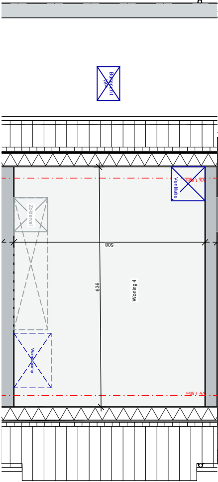
Zolderruimte
