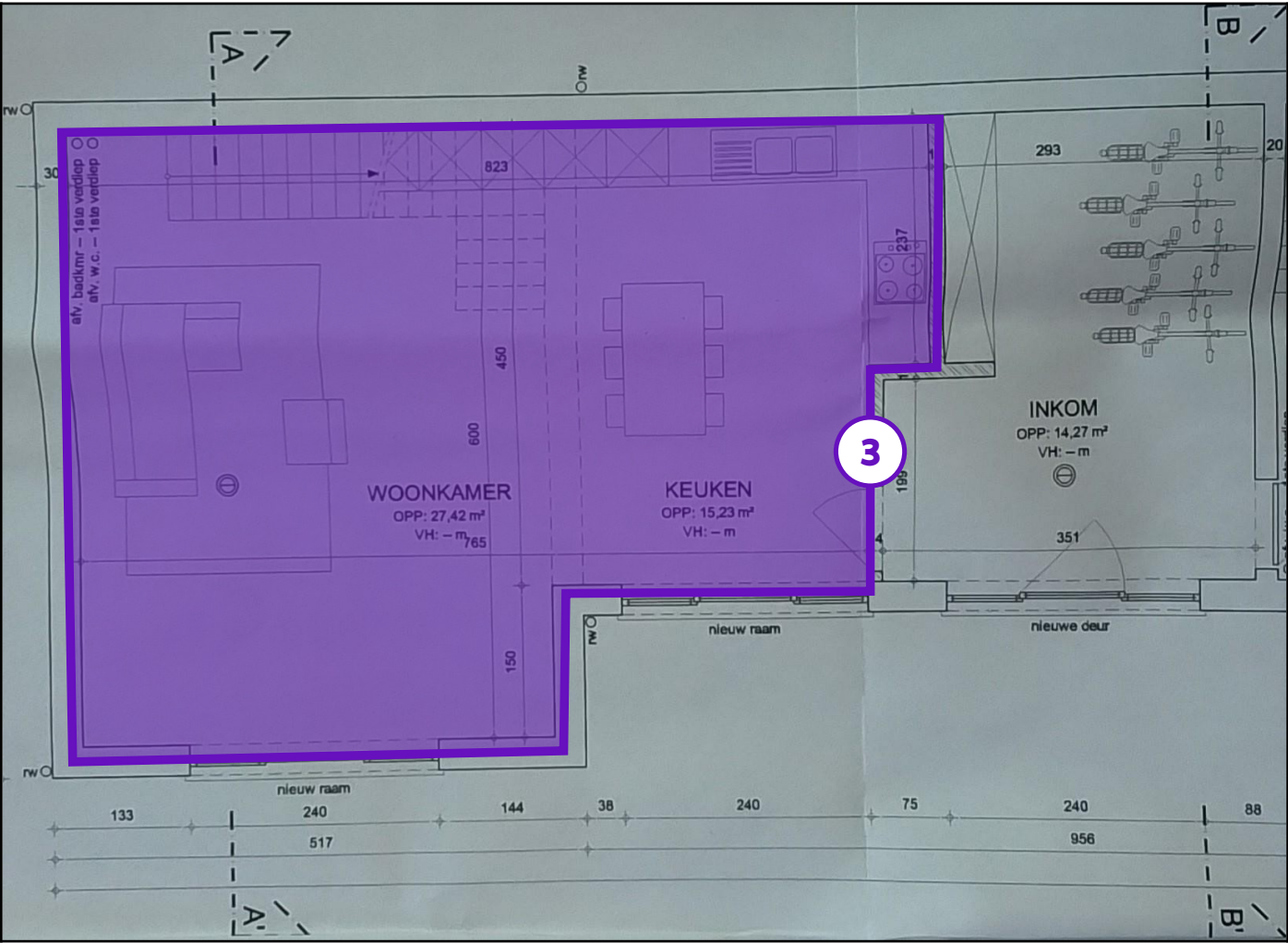
Legende van plan 1.3: Gelijkvloers : vals plafond
