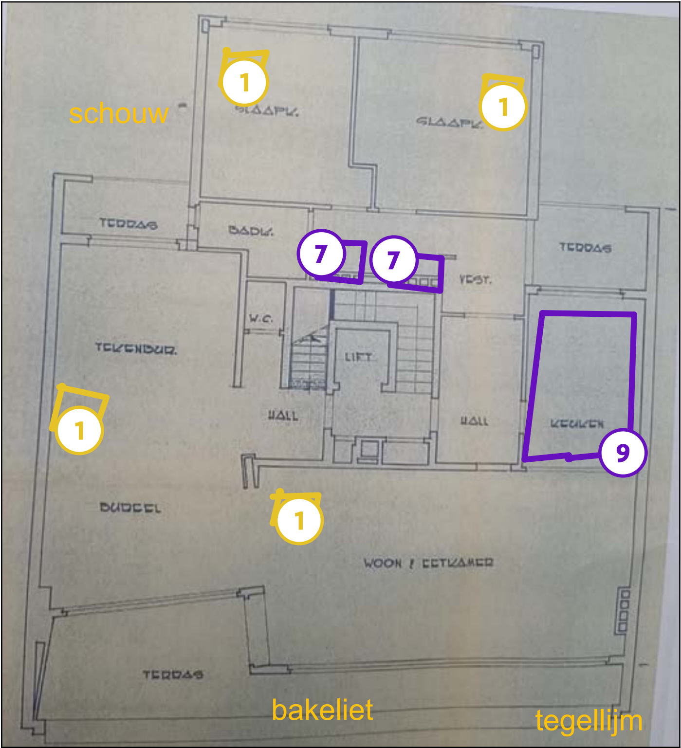
Legende van plan 1.3: plan appartement kopie kopie
