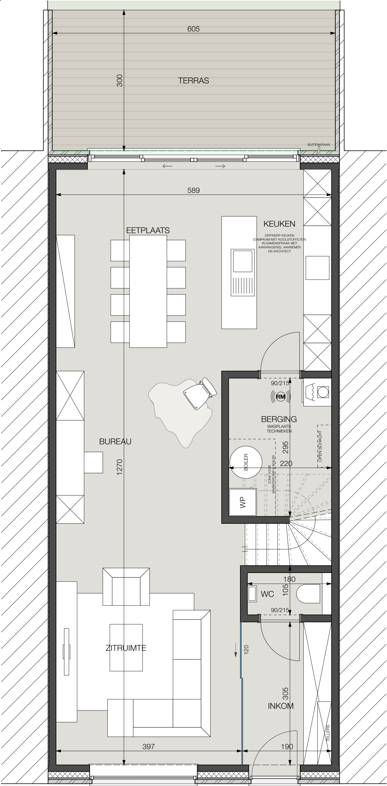
WONING 3: GRONDPLAN
