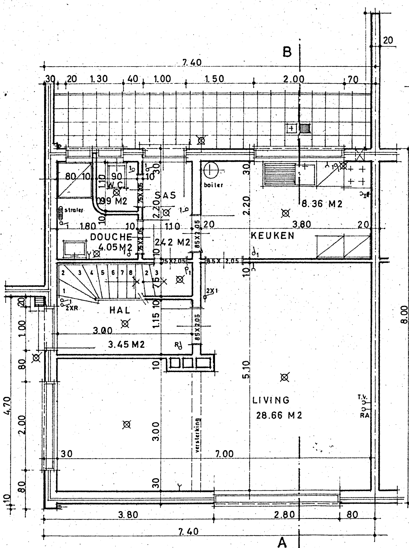
GELIJKVLOERS
