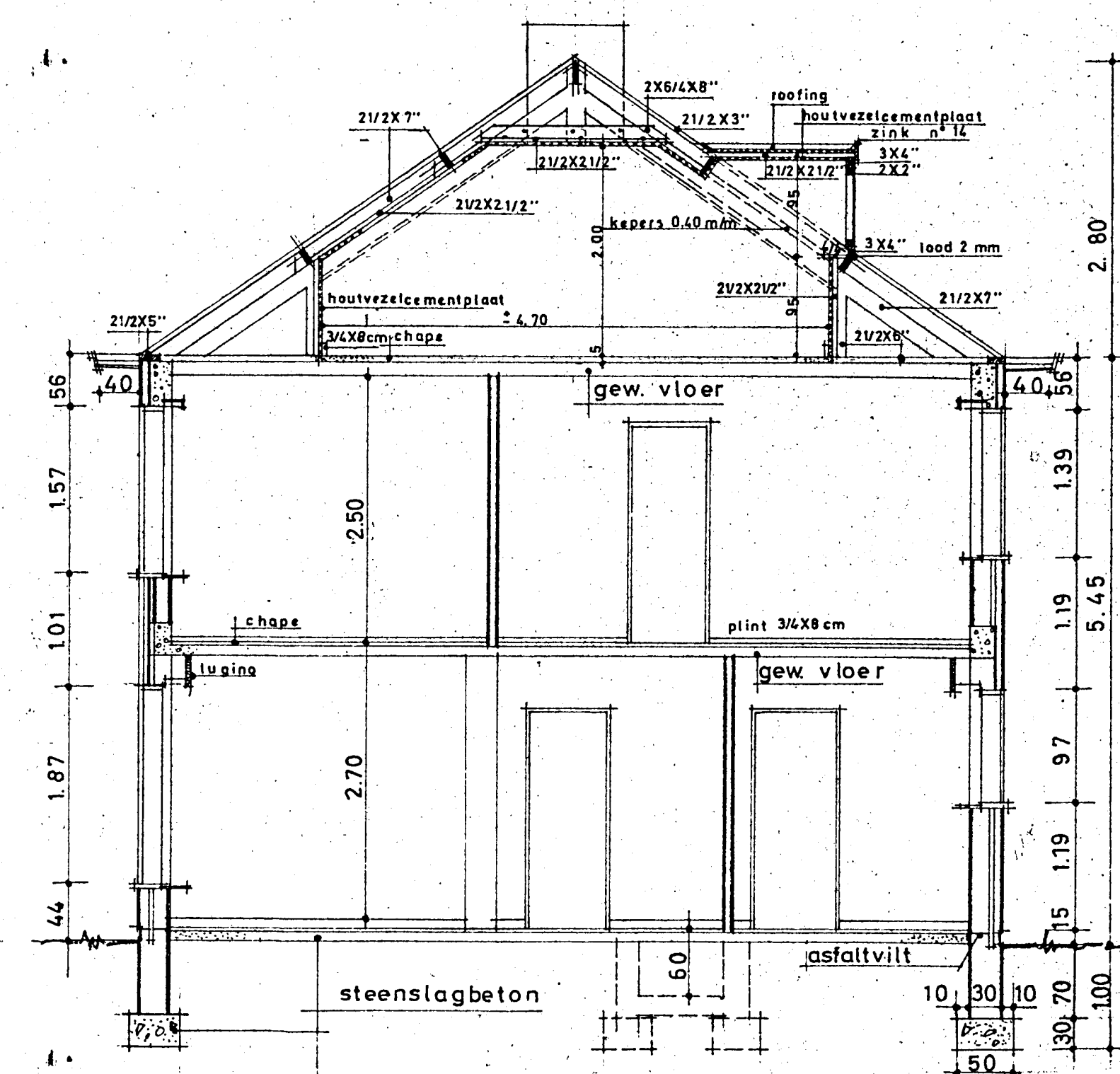
DOORSNEDE: A-B.
