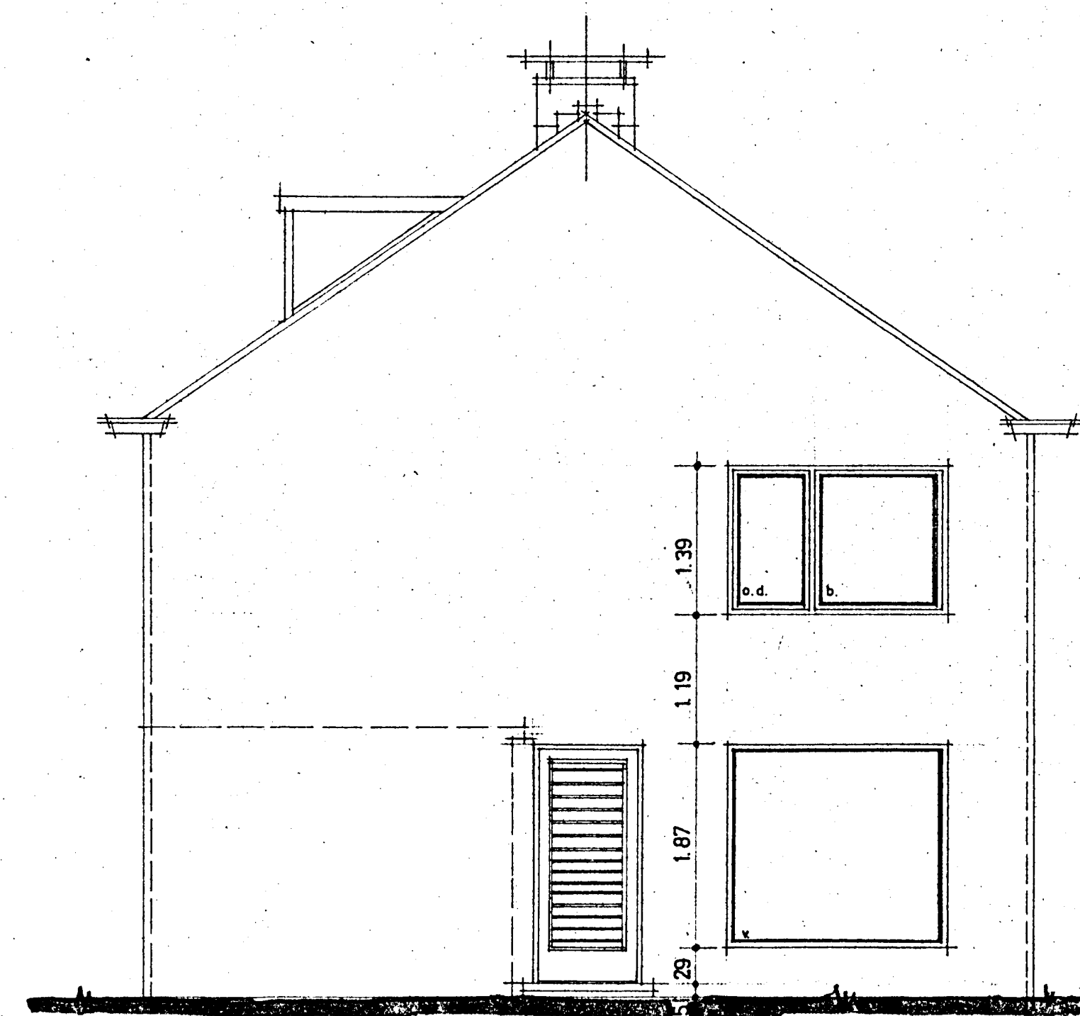
ZUGEVEL LINKS
