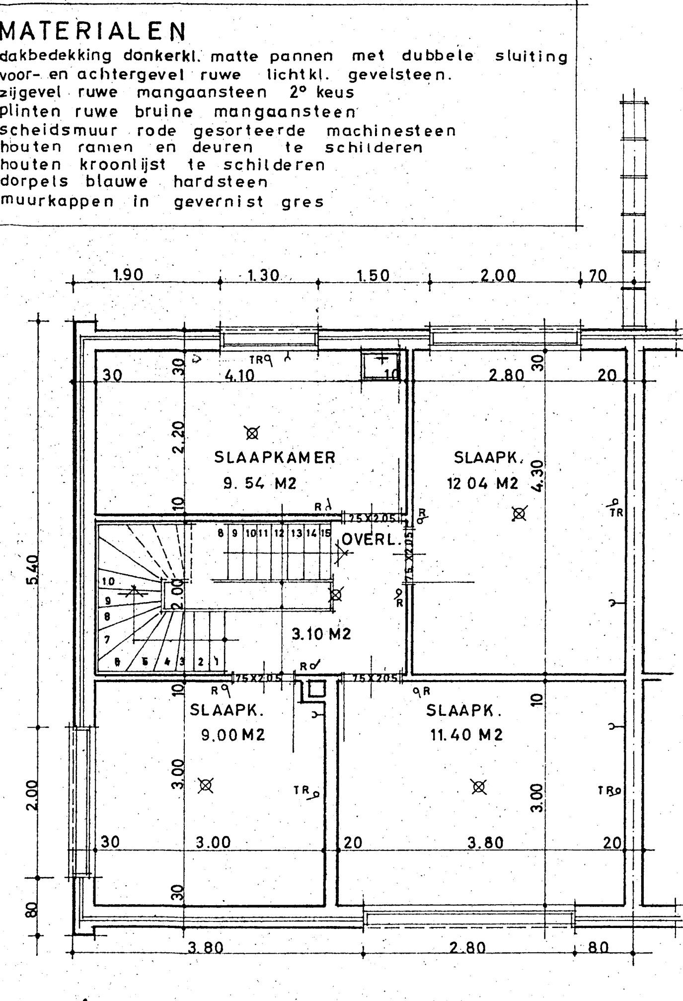
VERDIEPING
