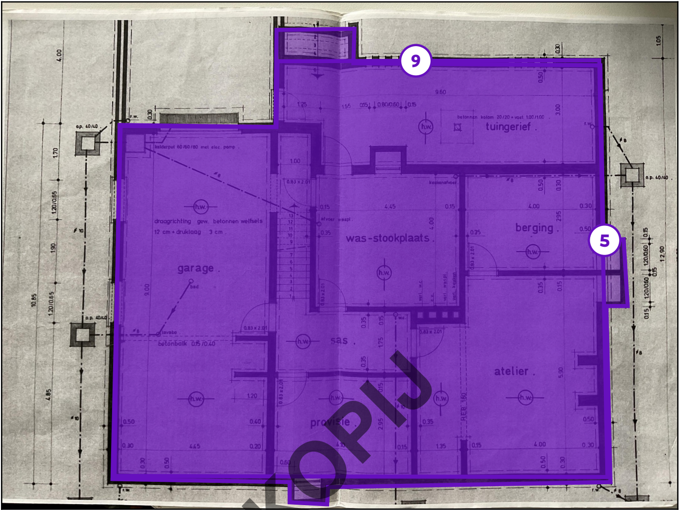
Legende van plan 1.5: Plan van de kelder
