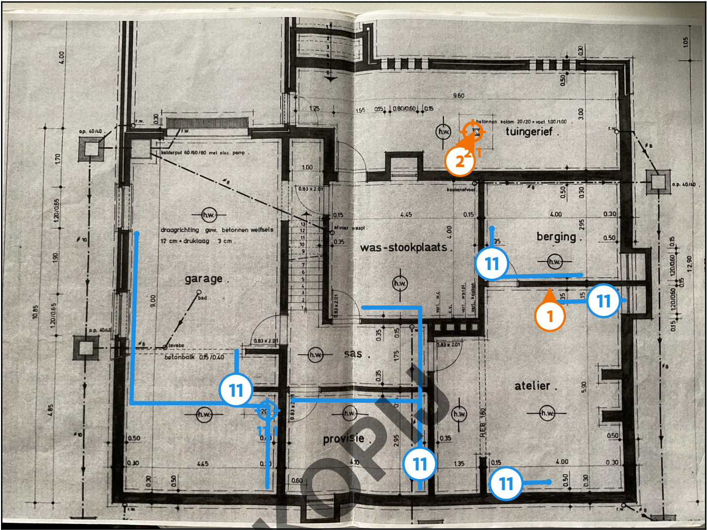
Legende van plan 1.4: Plan van de kelder
