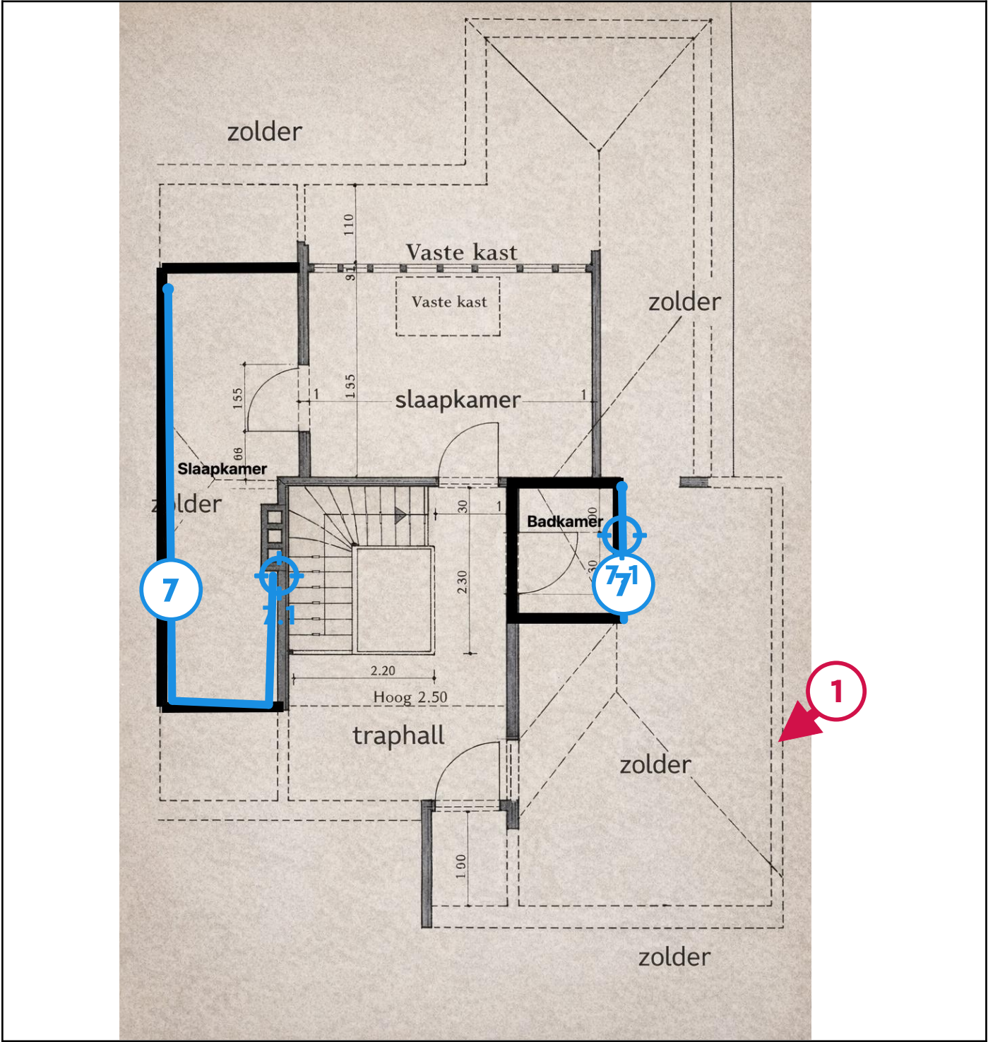
Legende van plan 1.5: Eerste verdieping
