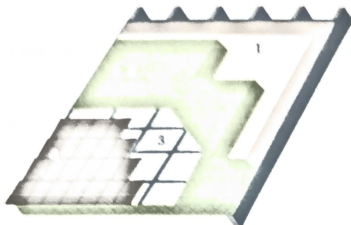
1. Dampscherm | 2. Isolatie | 3. Onderdak | 4. Dakbekleding
