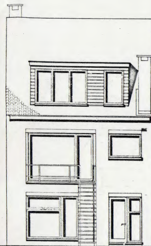
Achtergevel.
