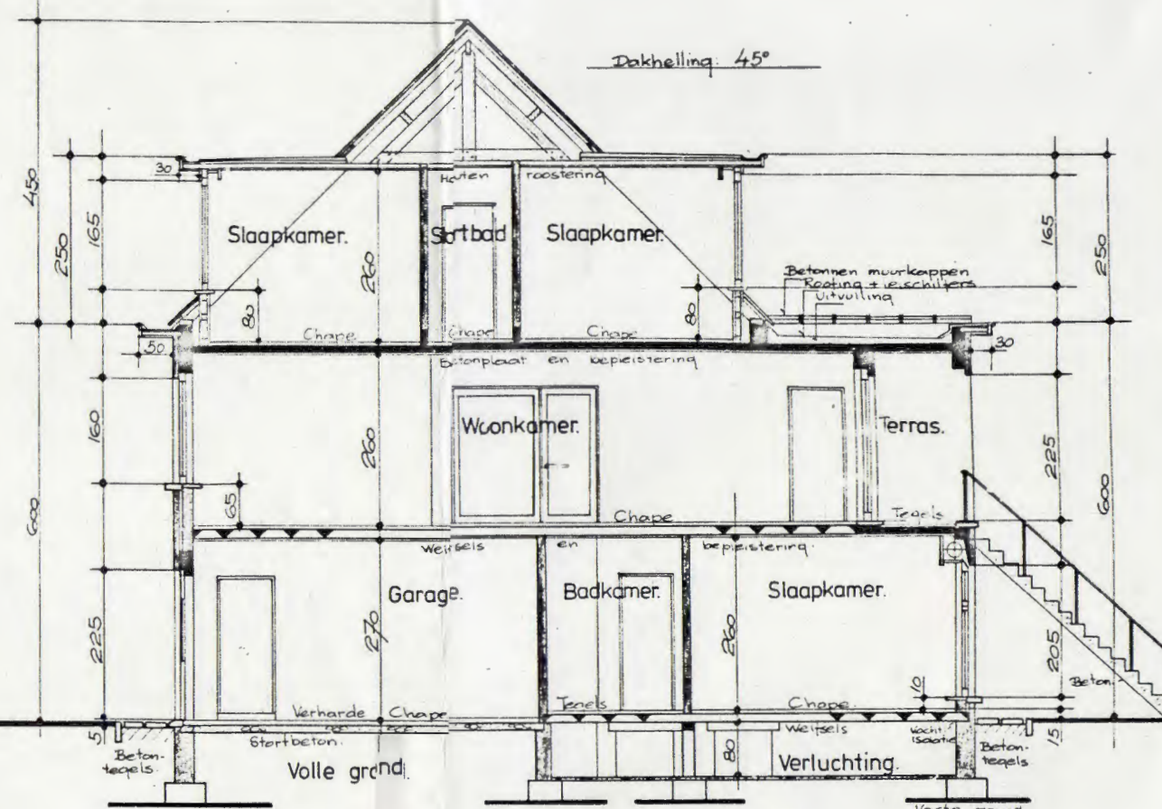
Doorsnede: A-B.
