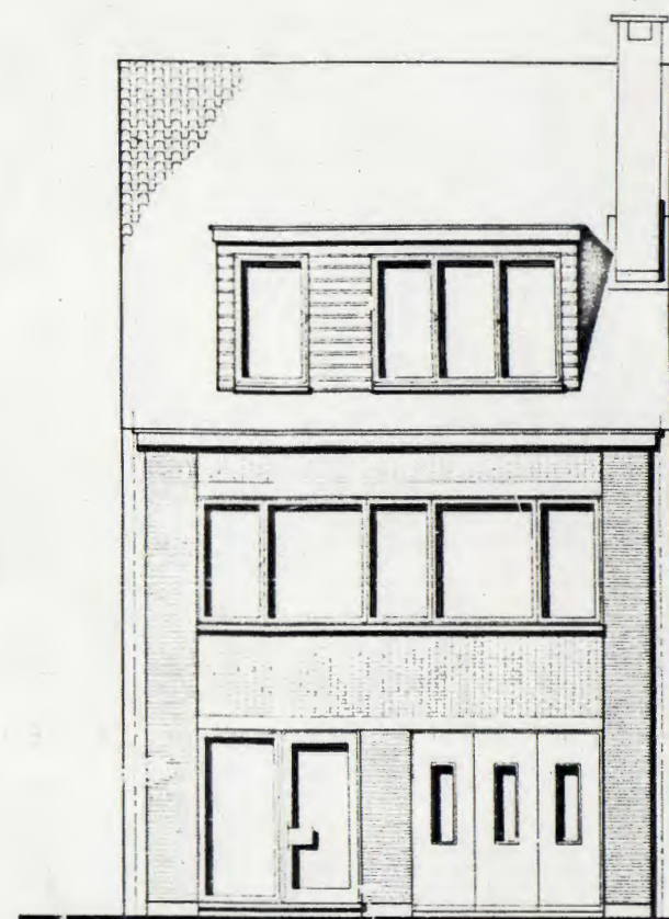
Voorgevel.
