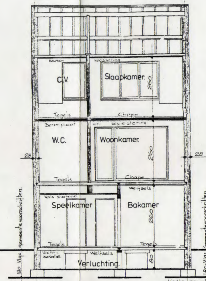
Doorsnede: C-D.
