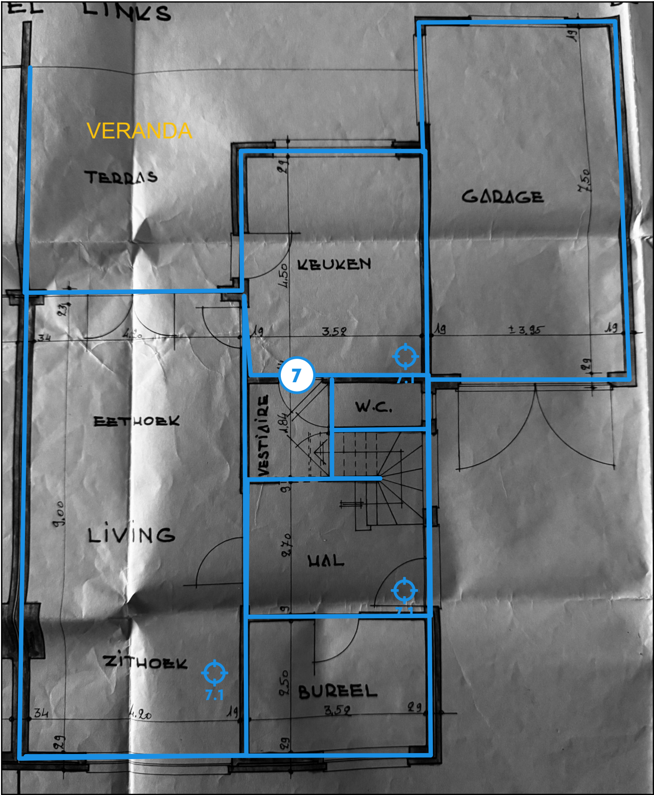
Legende van plan 1.3: Verdieping V0
