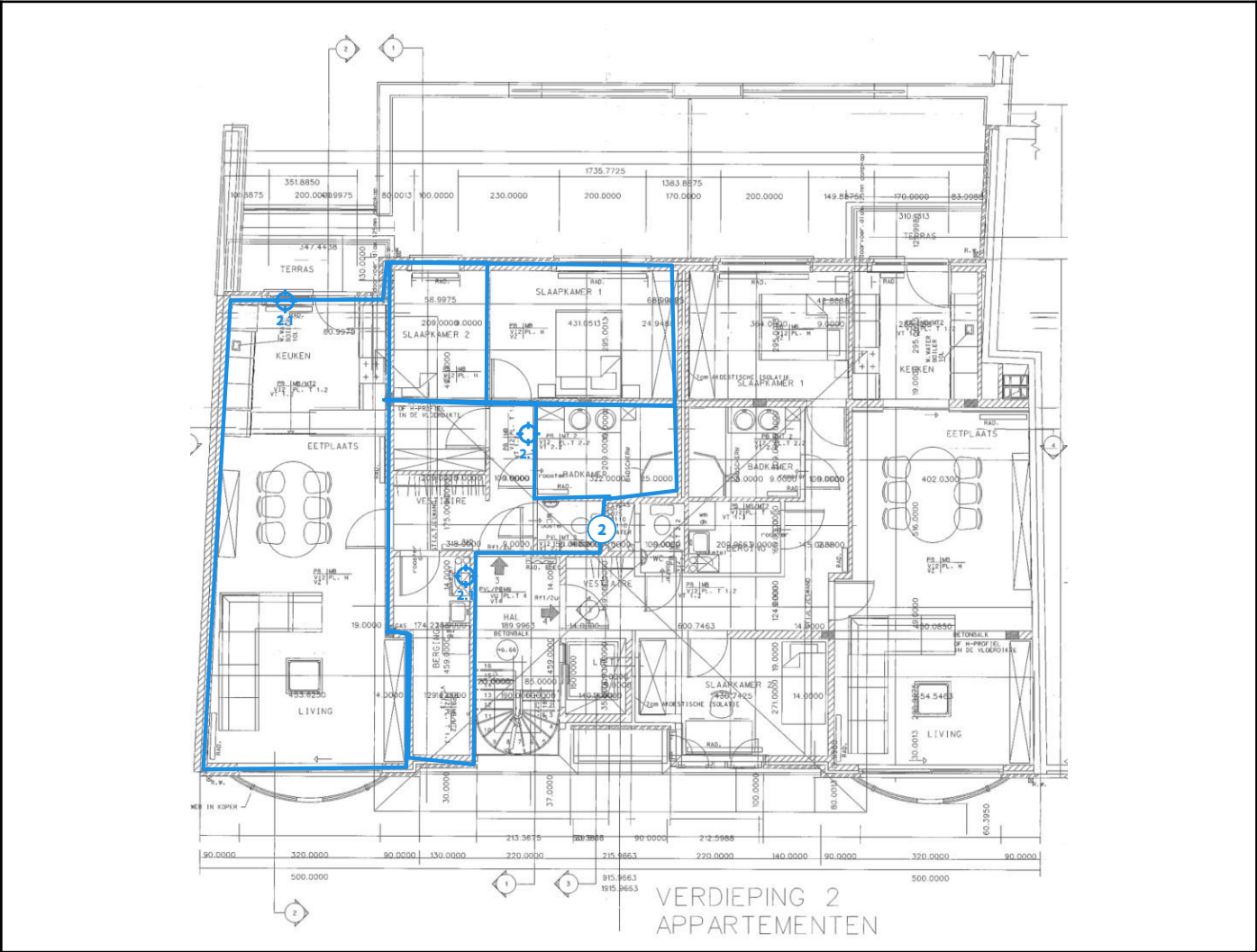
Legende van plan 1.1: plan verdieping 2
