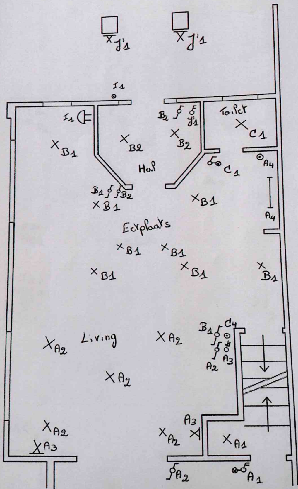
Grondplan benedenverdieping
