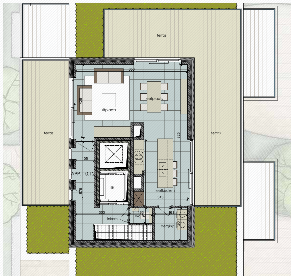
VERDIEPING 2
