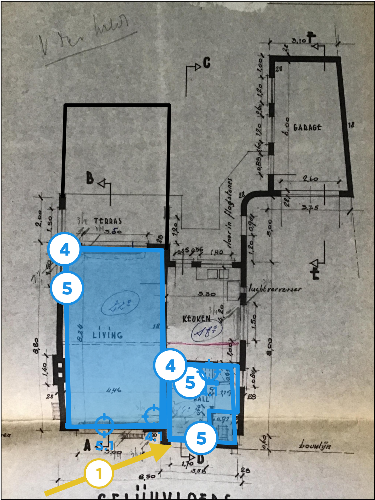
Legende van plan 1.2: Hoofdegebouw plan gelijkvloers
