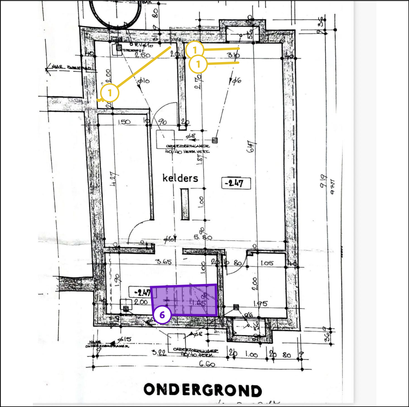
Legende van plan 1.2: Plan kelder
