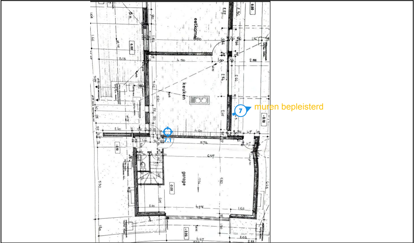
Legende van plan 1.8: Plan Gelijkvloers
