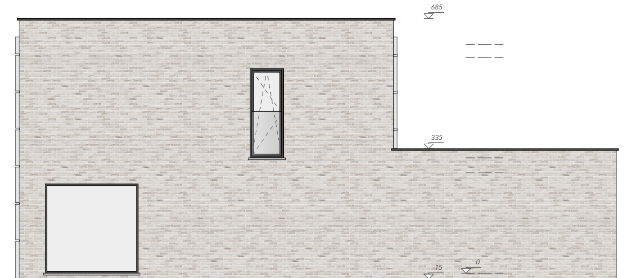
aanzicht zijgevel
