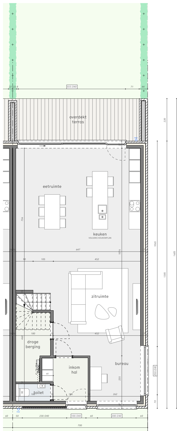
grondplan gelijkvloers
