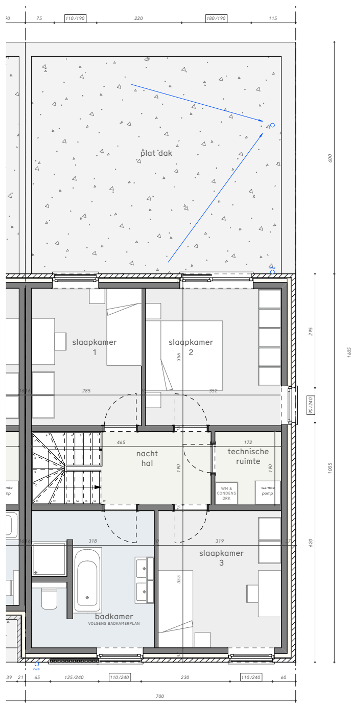
grondplan verdieping
