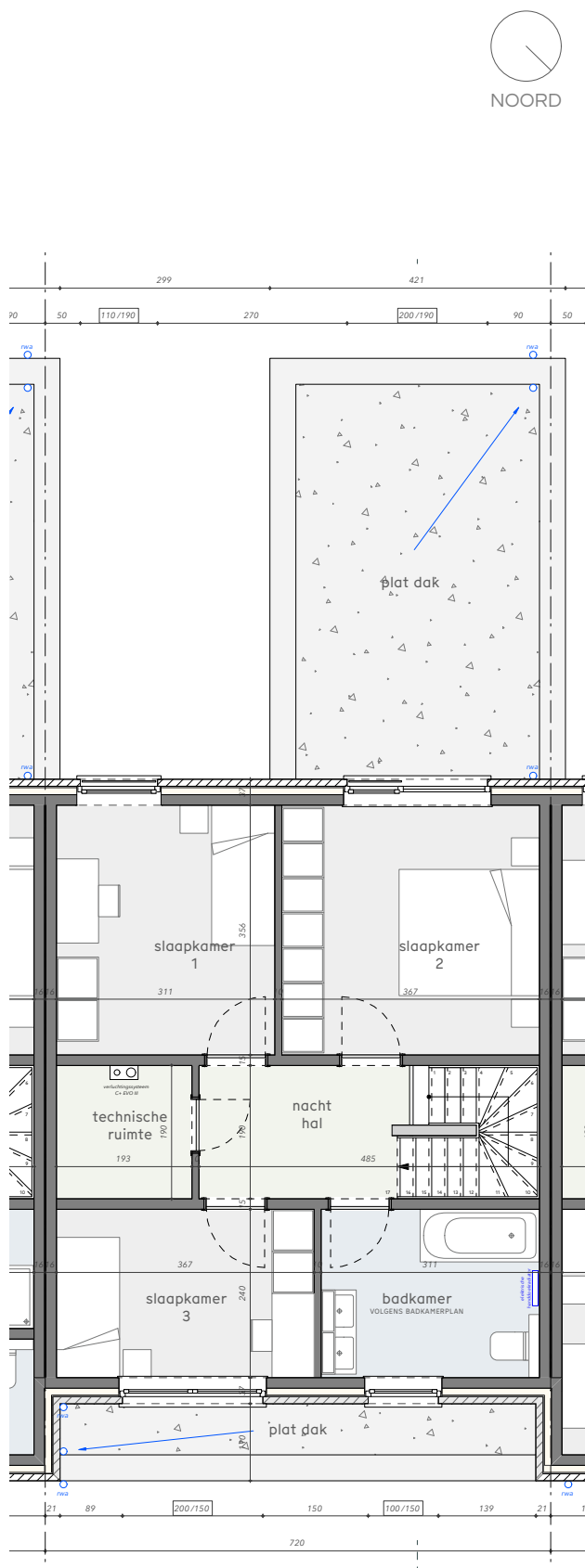
grondplan verdieping
