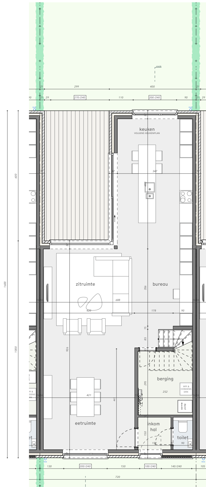
grondplan gelijkvloers
