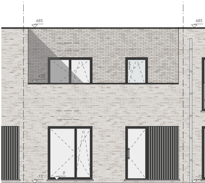
aanzicht voorgevel
