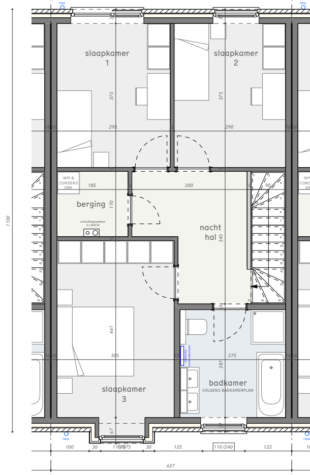
grondplan verdieping
