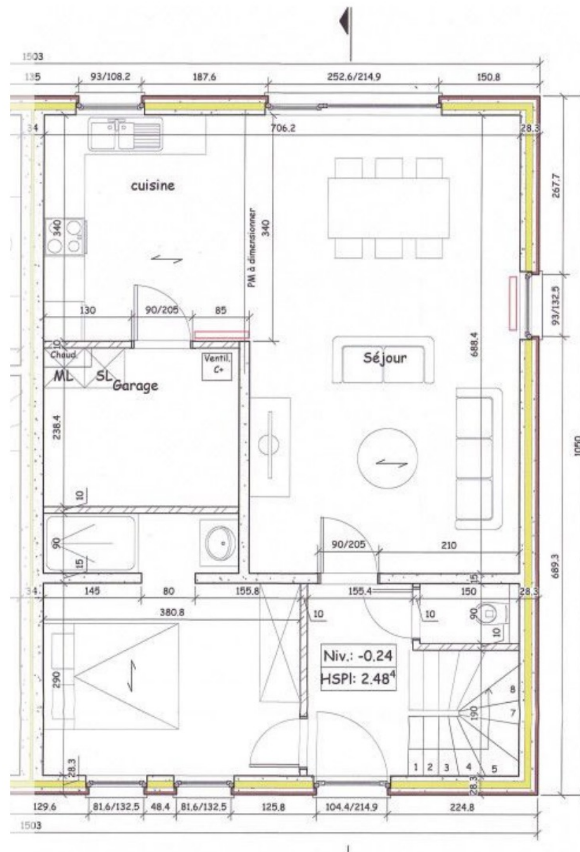
Rez-de-chaussée
