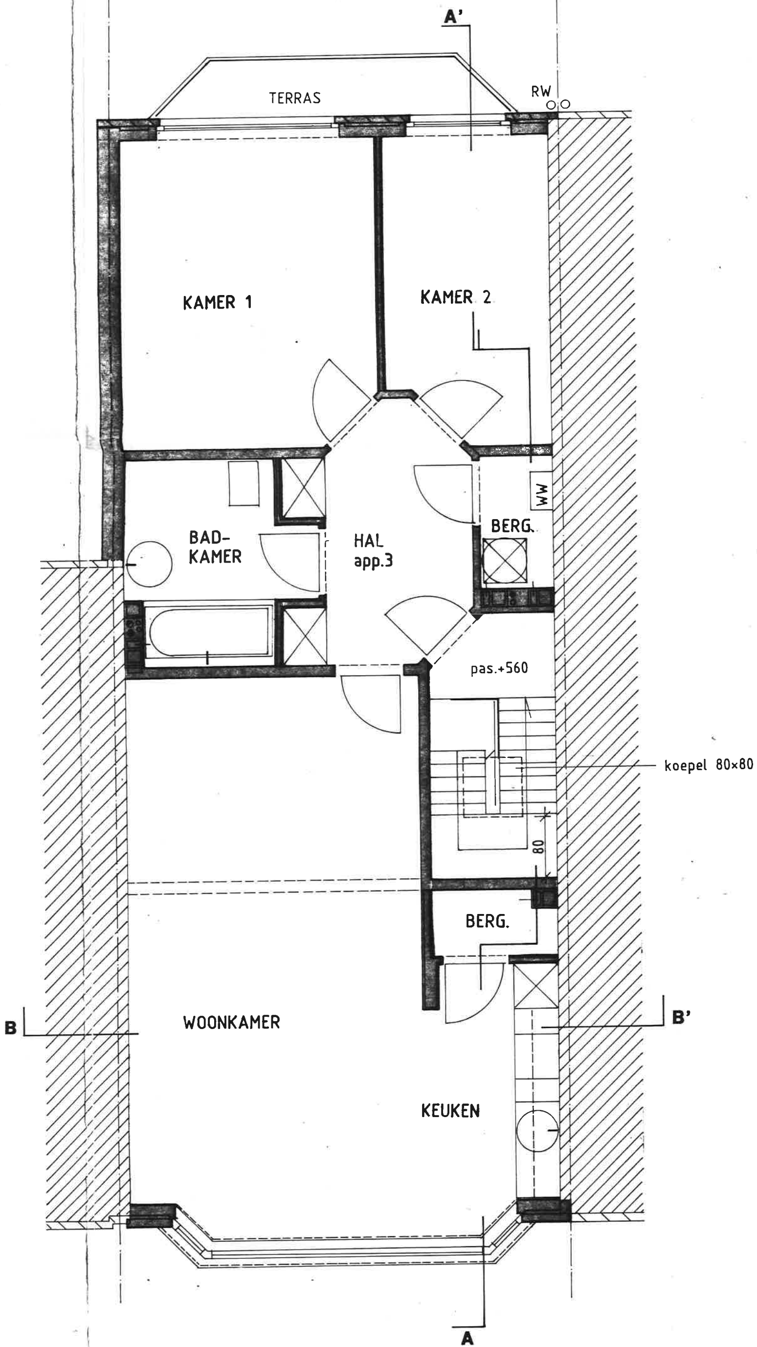
2° VERDIEPING
