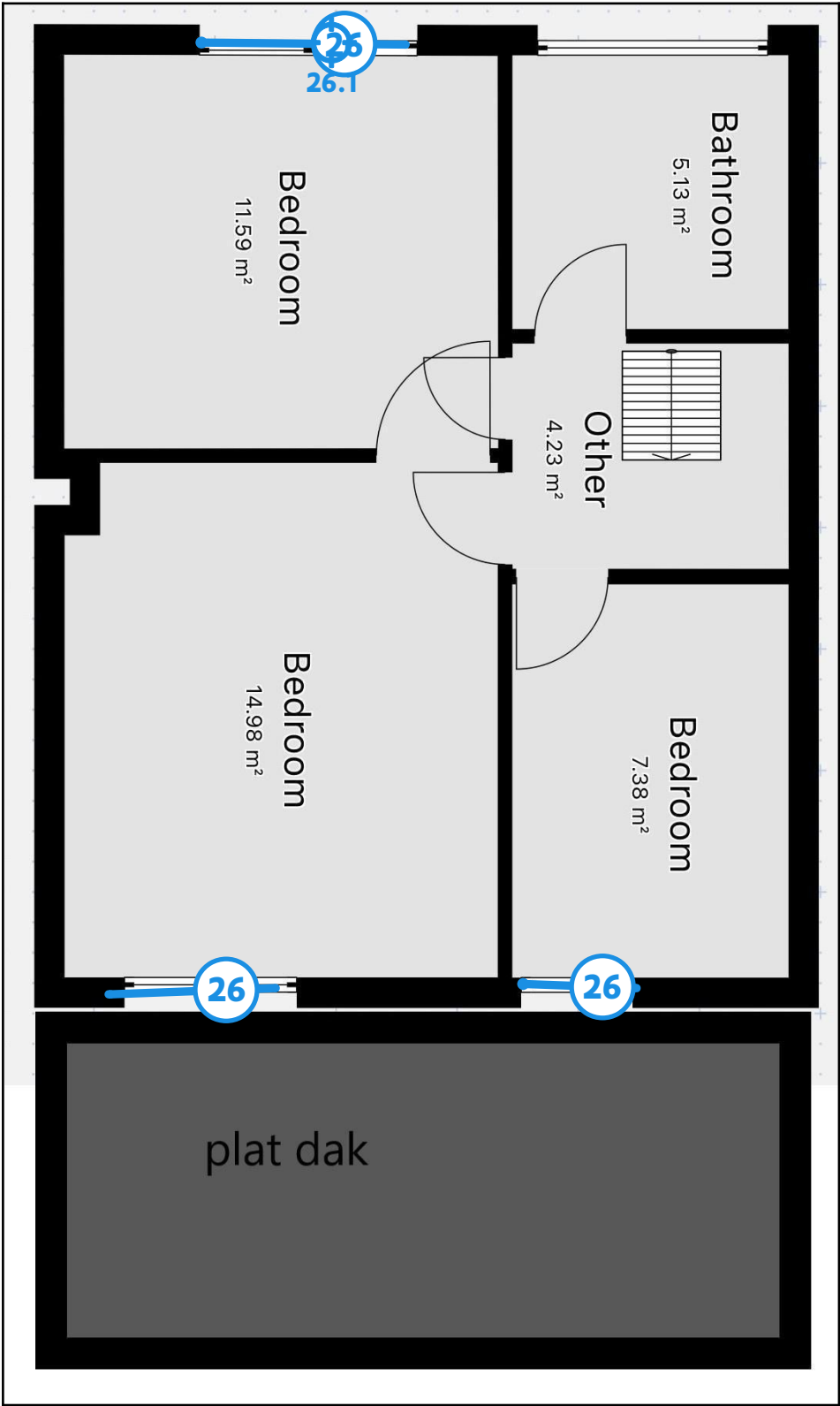
Legende van plan 1.14: Verdieping 2 woning
