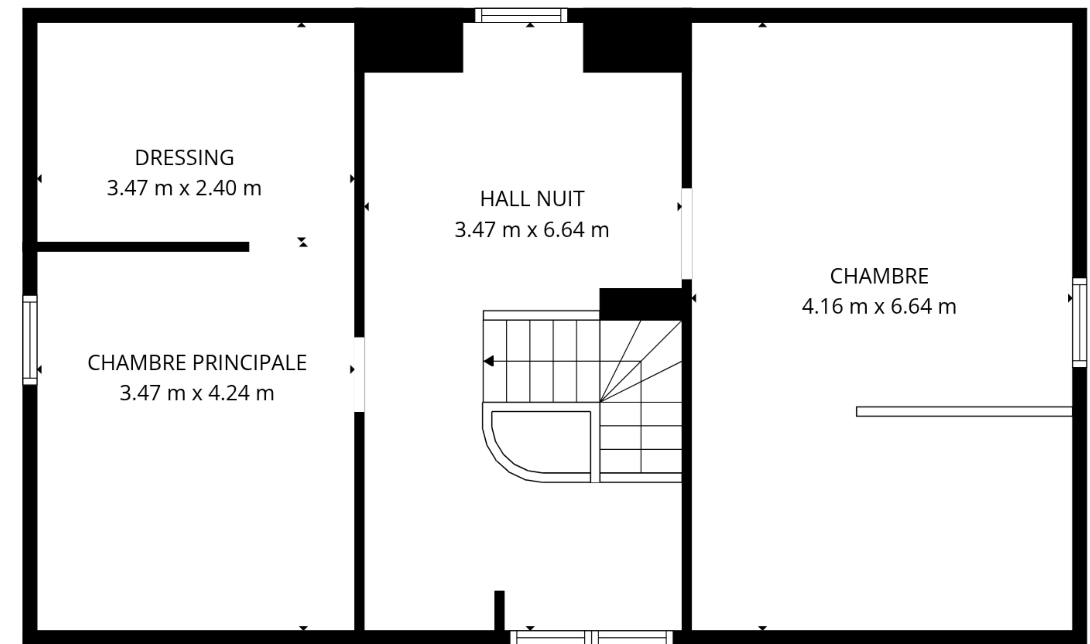
1er étage
