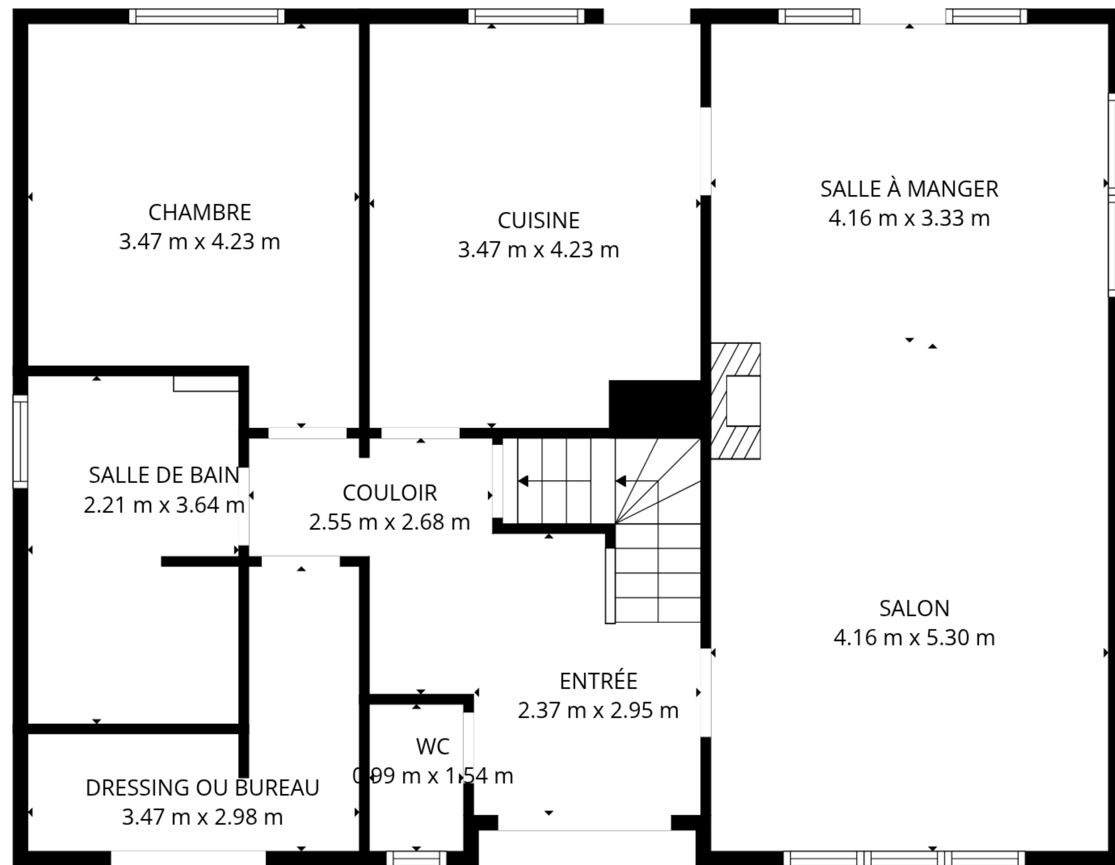
Rez-de-chaussée
