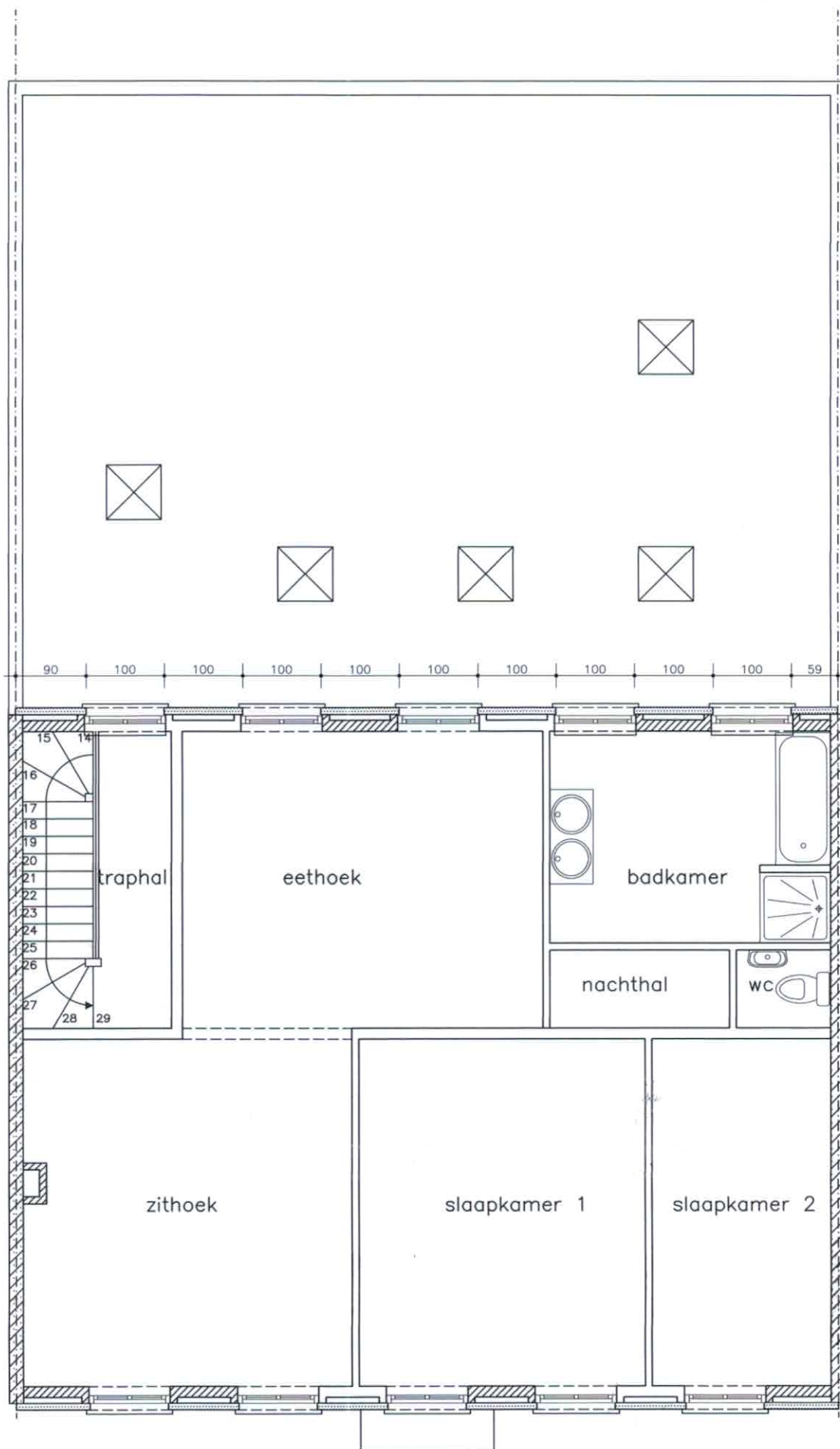
VERDIEPING ongewijzigd SCHAAL 1/50
