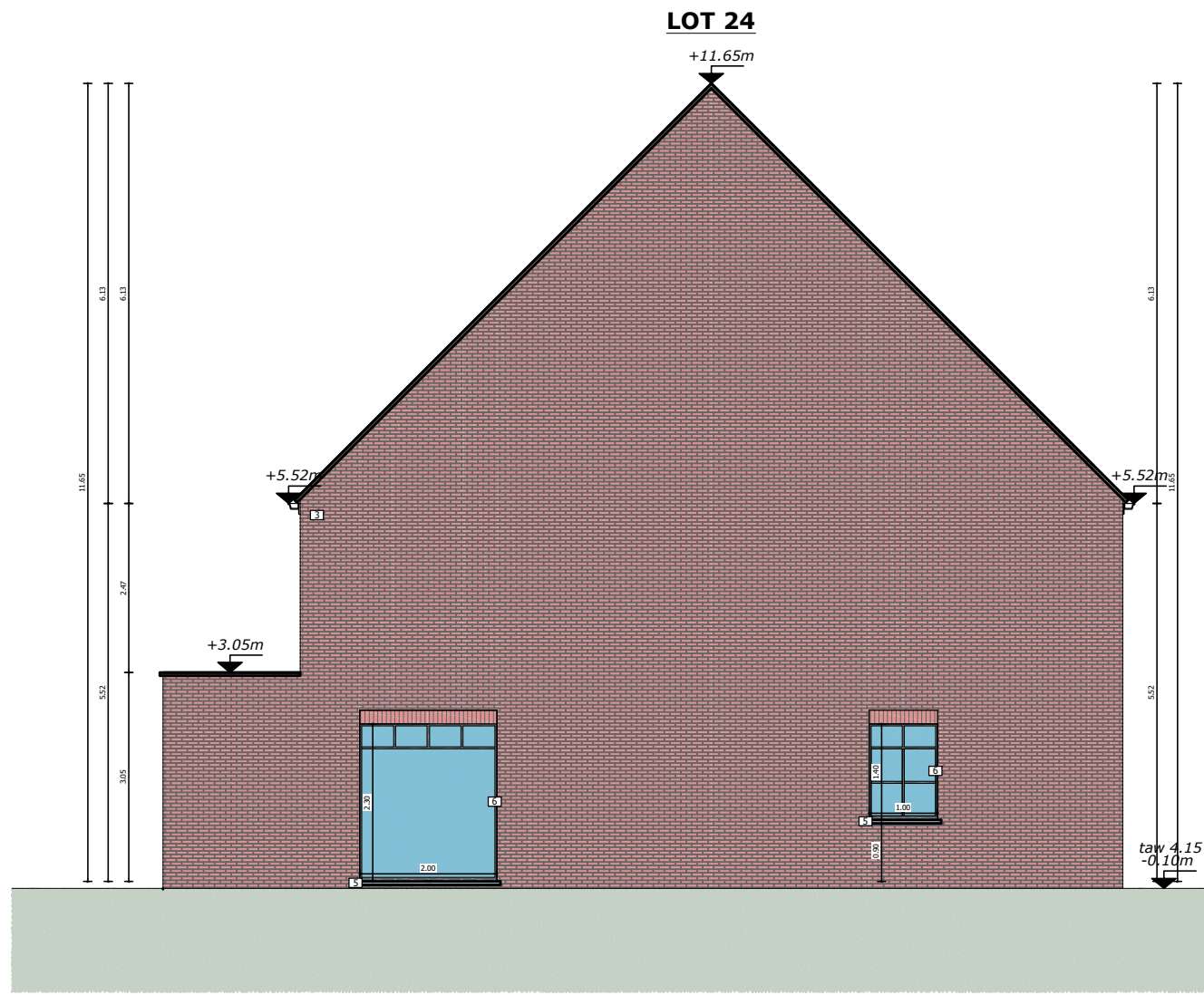
Zijgevel links
