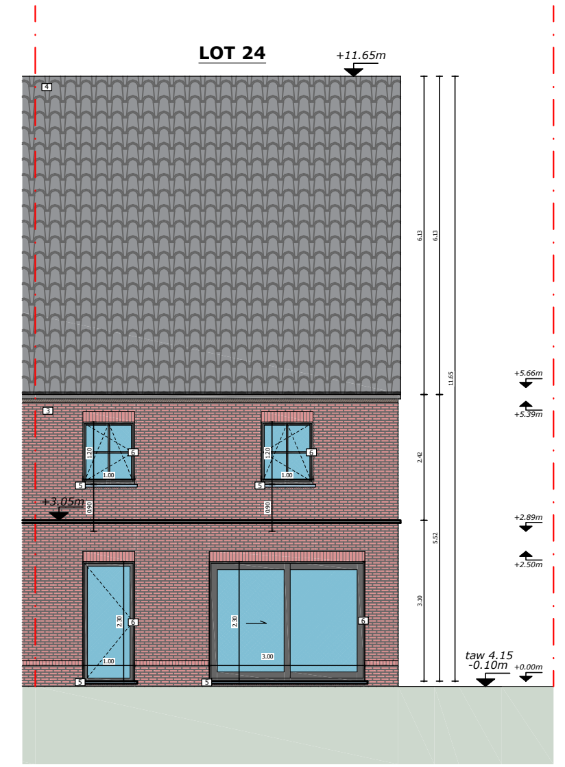
Achtergevel
