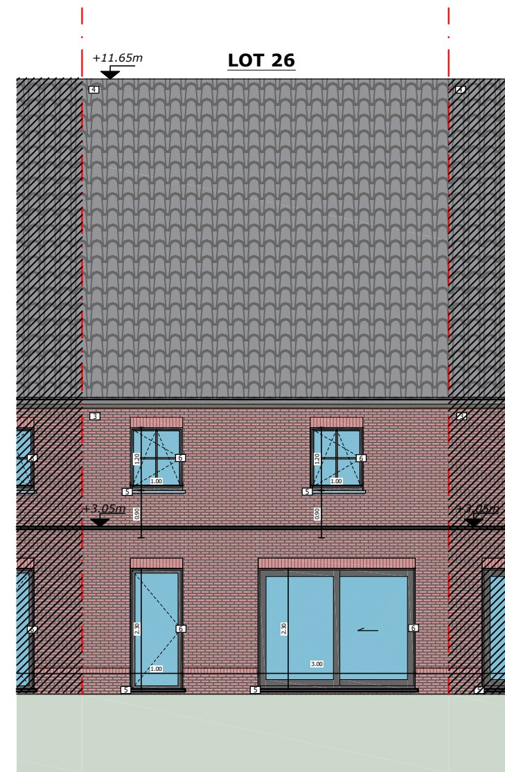
Achtergevel
