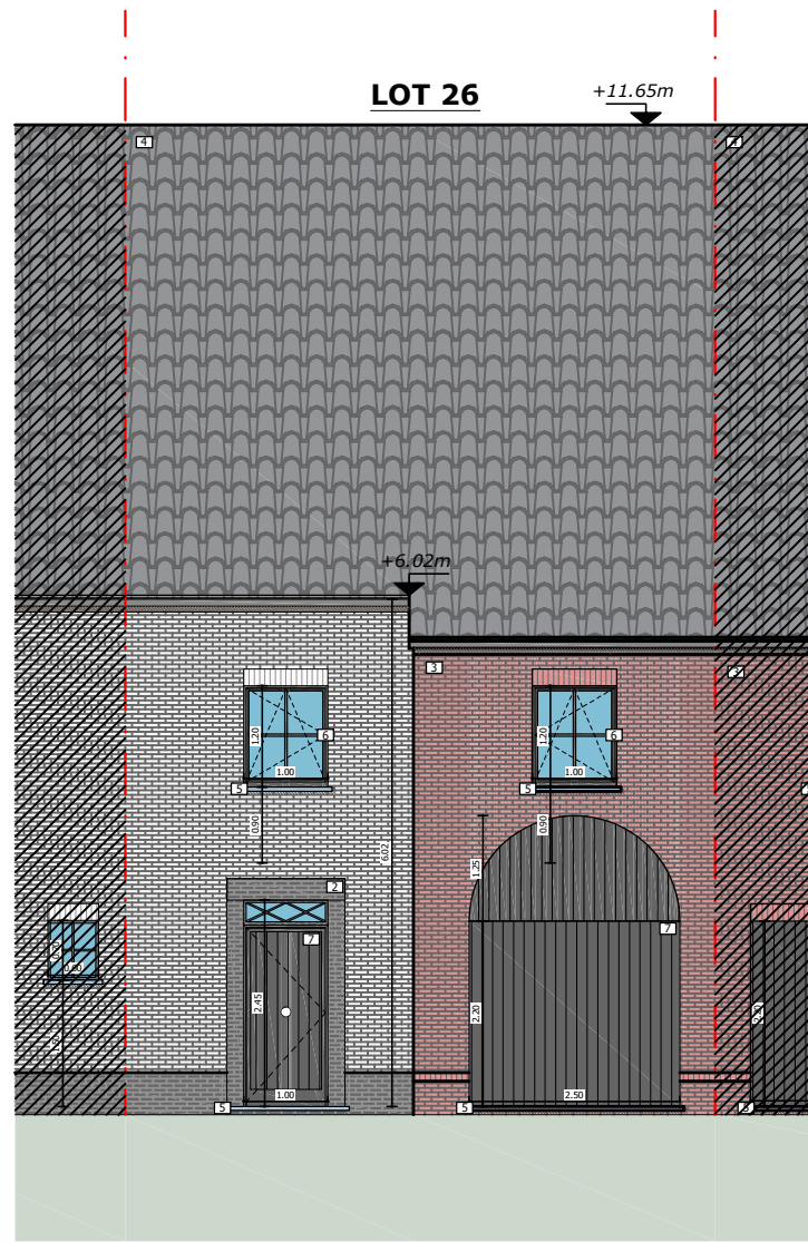
Voorgevel
