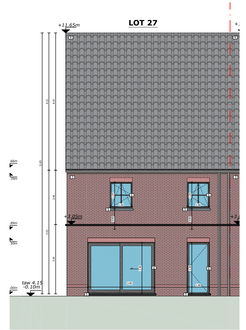
Achtergevel
