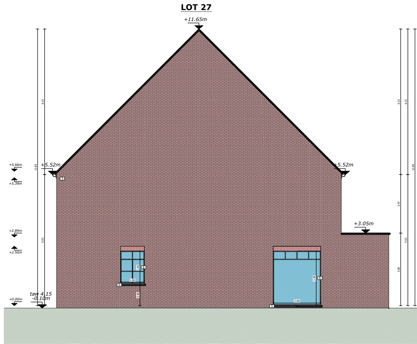
Zijgevel rechts
