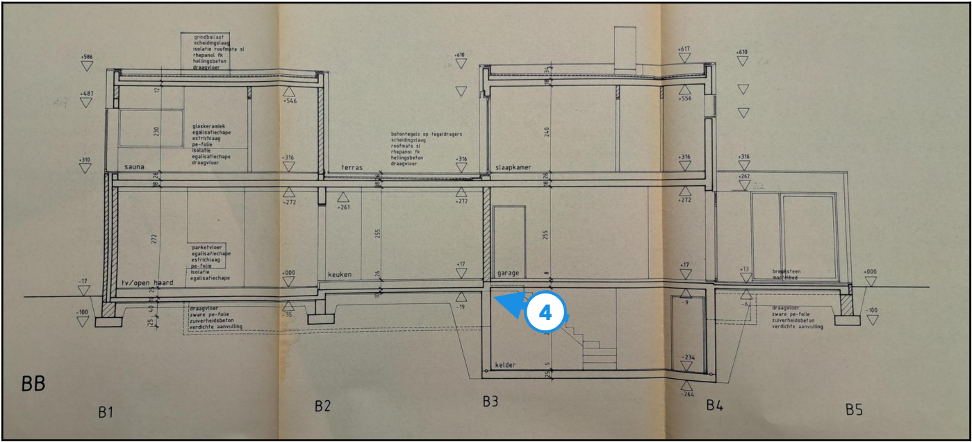
Legende van plan 1.4: leidingisolatie
