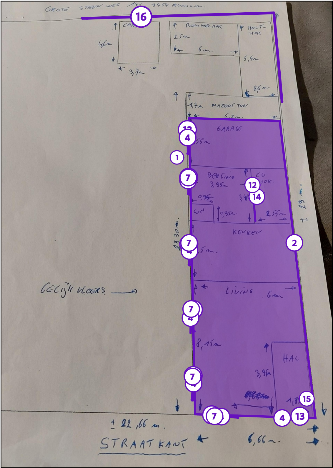
Legende van plan 1.2: Gelijkvloers - Bronfiches & adviezen
