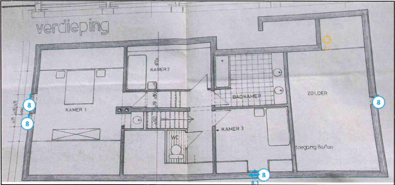
Legende van plan 1.3: Plan Bovenverdieping
