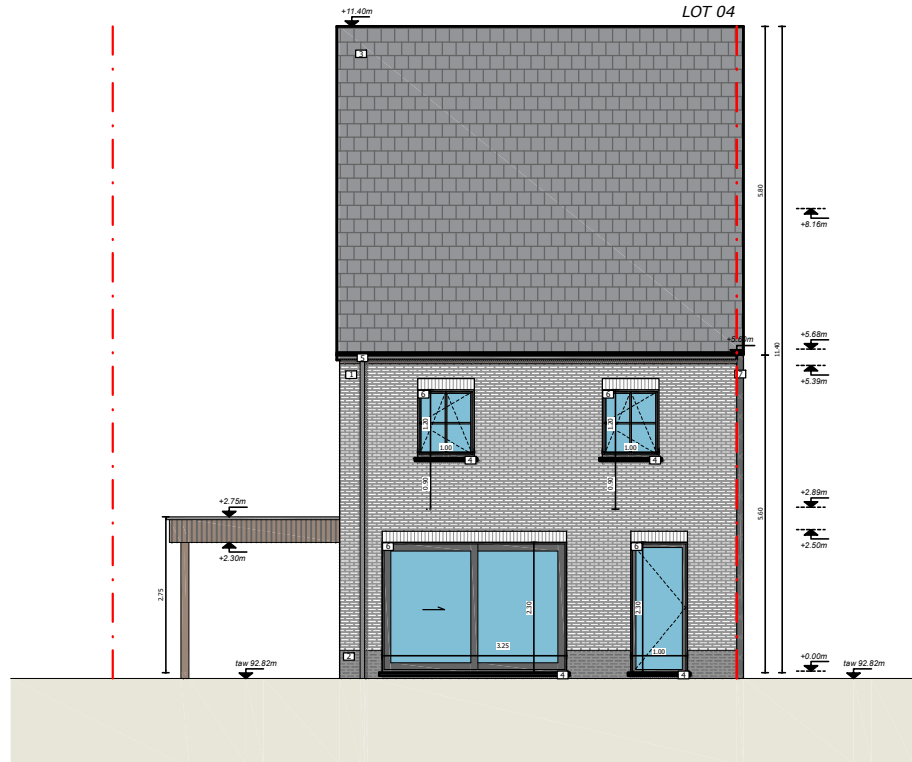
Achtergevel
