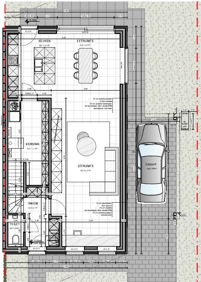
Gelijkvloers
