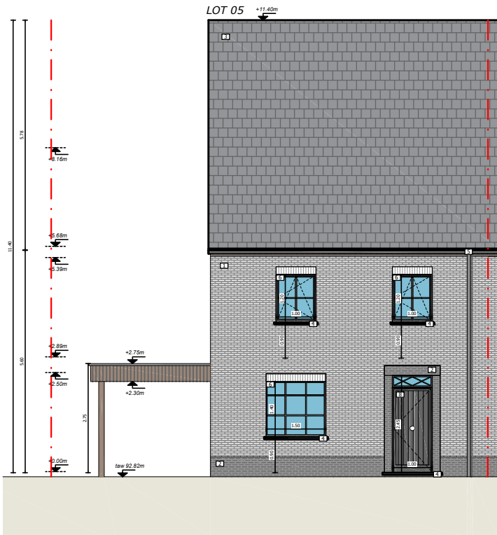
Voorgevel
