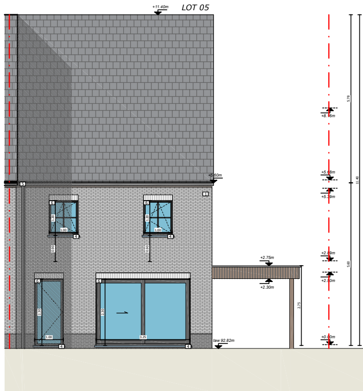
Achtergevel
