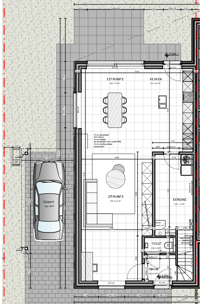
Gelijkvloers
