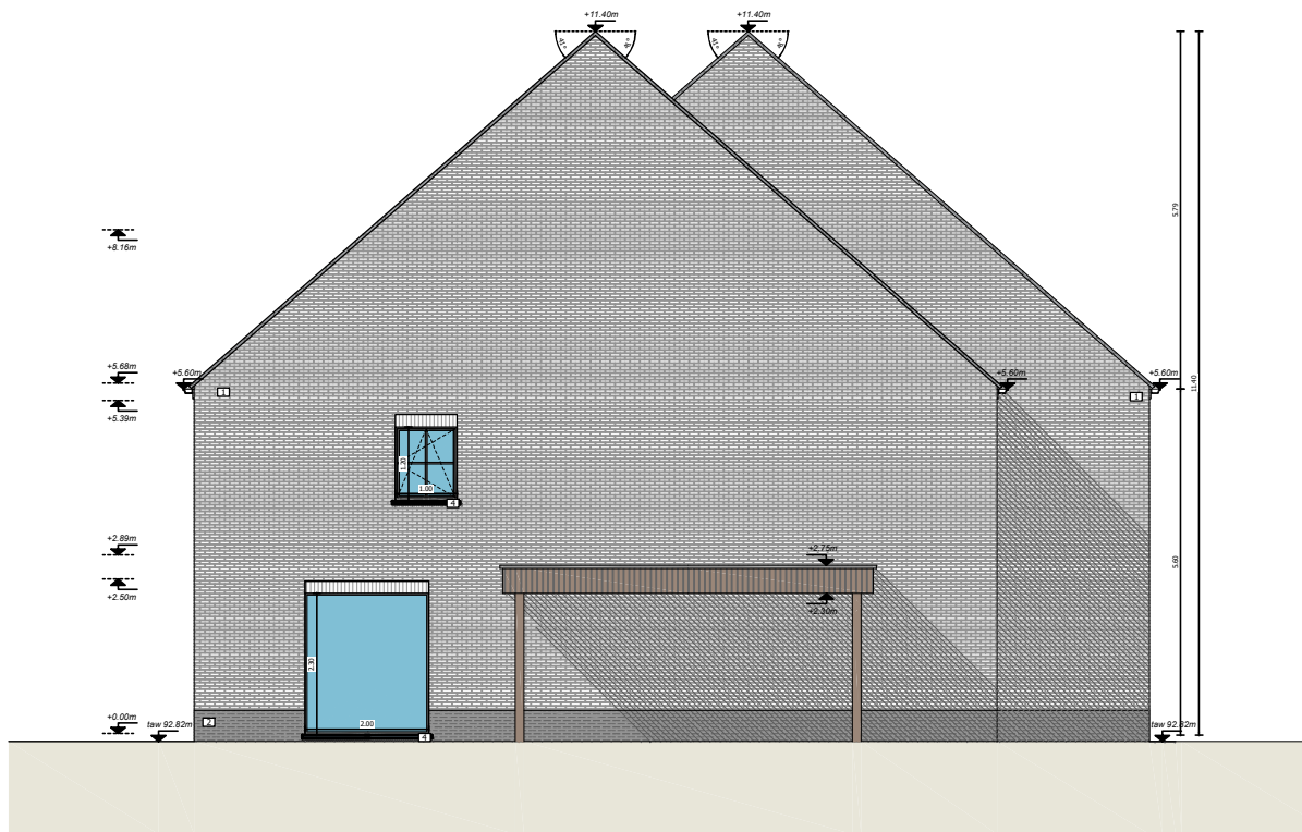
Zijgevel links
