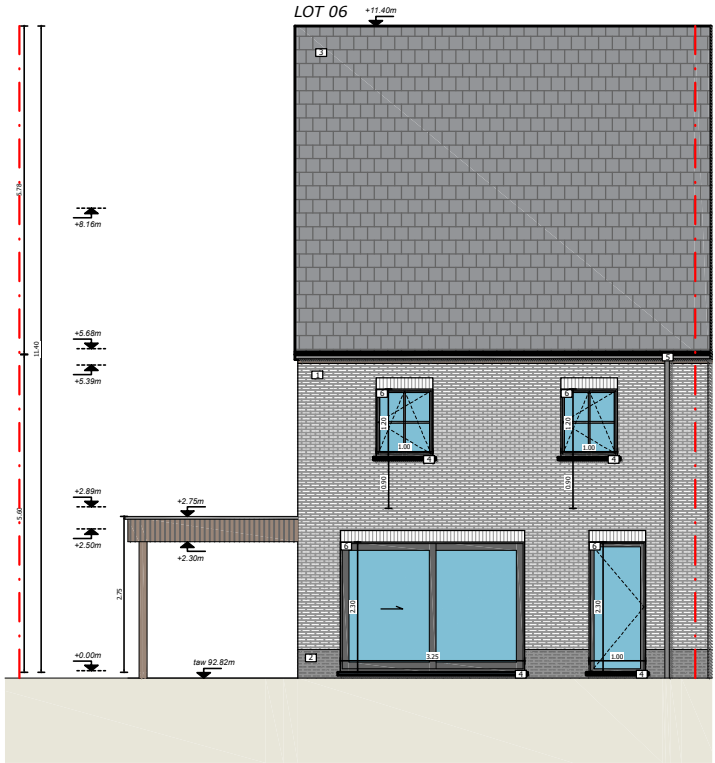
Achtergevel
