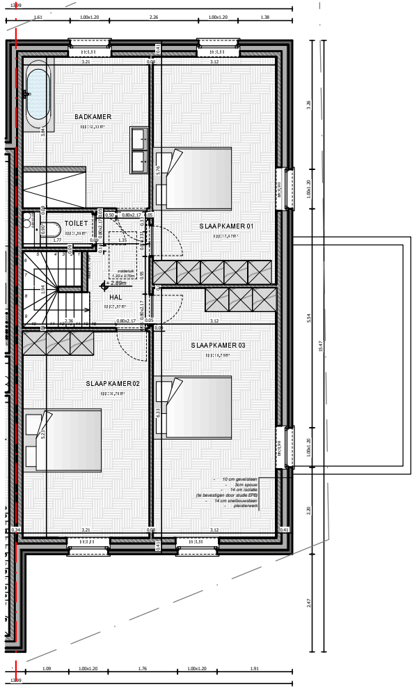
1e Verdieping
