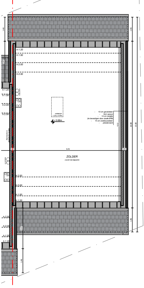
2e Verdieping
