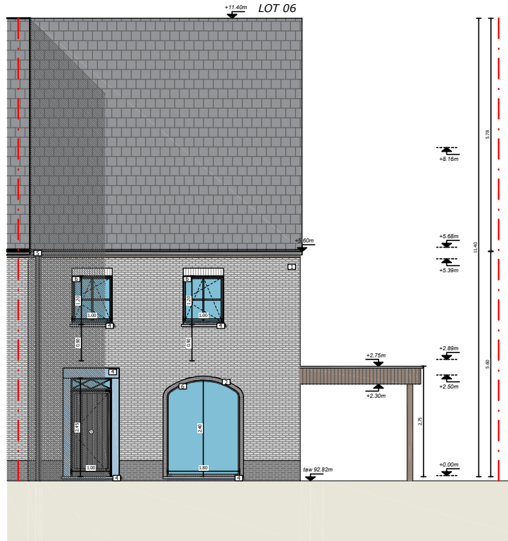
Voorgevel
