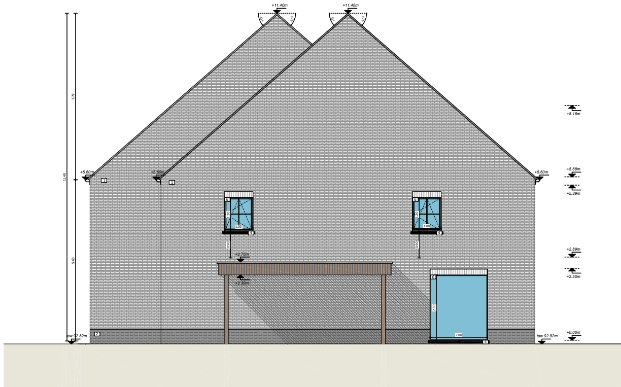
Zijgevel links
