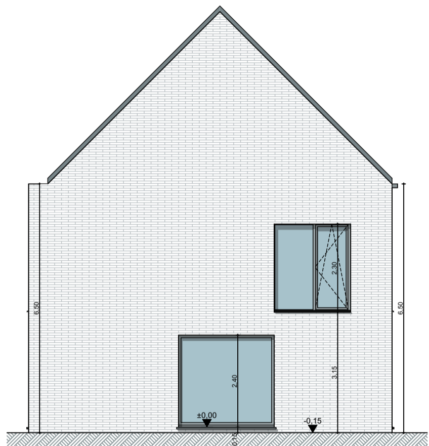
WONING 1: zijgevel links 1:100
