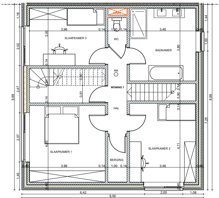
WONING 1: plan 1e verdieping 1:100
