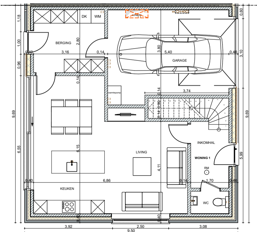
WONING 1: plan gelijkvloers 1:100
