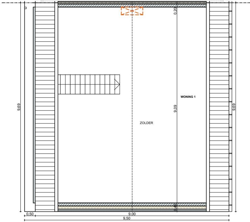
WONING 1: plan 2e verdieping 1:100
