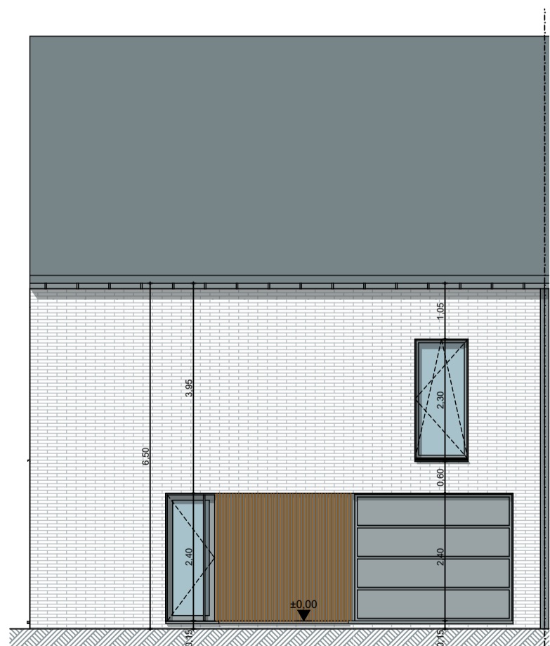
WONING 1: voorgevel 1:100
