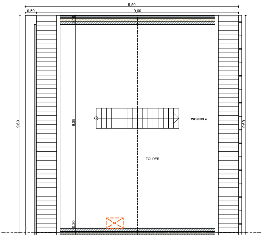
WONING 4: plan 2e verdieping 1:100
