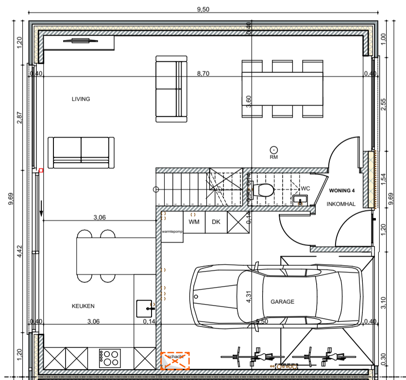
WONING 4: plan gelijkvloers 1:100
