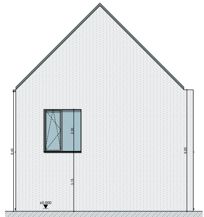
WONING 4: zijgevel rechts 1:100
