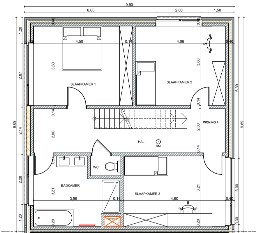
WONING 4: plan 1e verdieping 1:100
