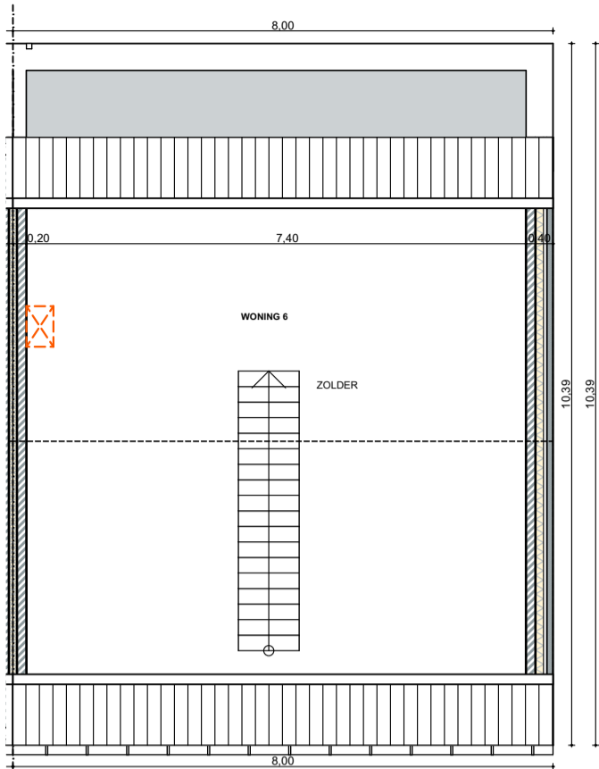
WONING 6: plan 2e verdieping 1:100
