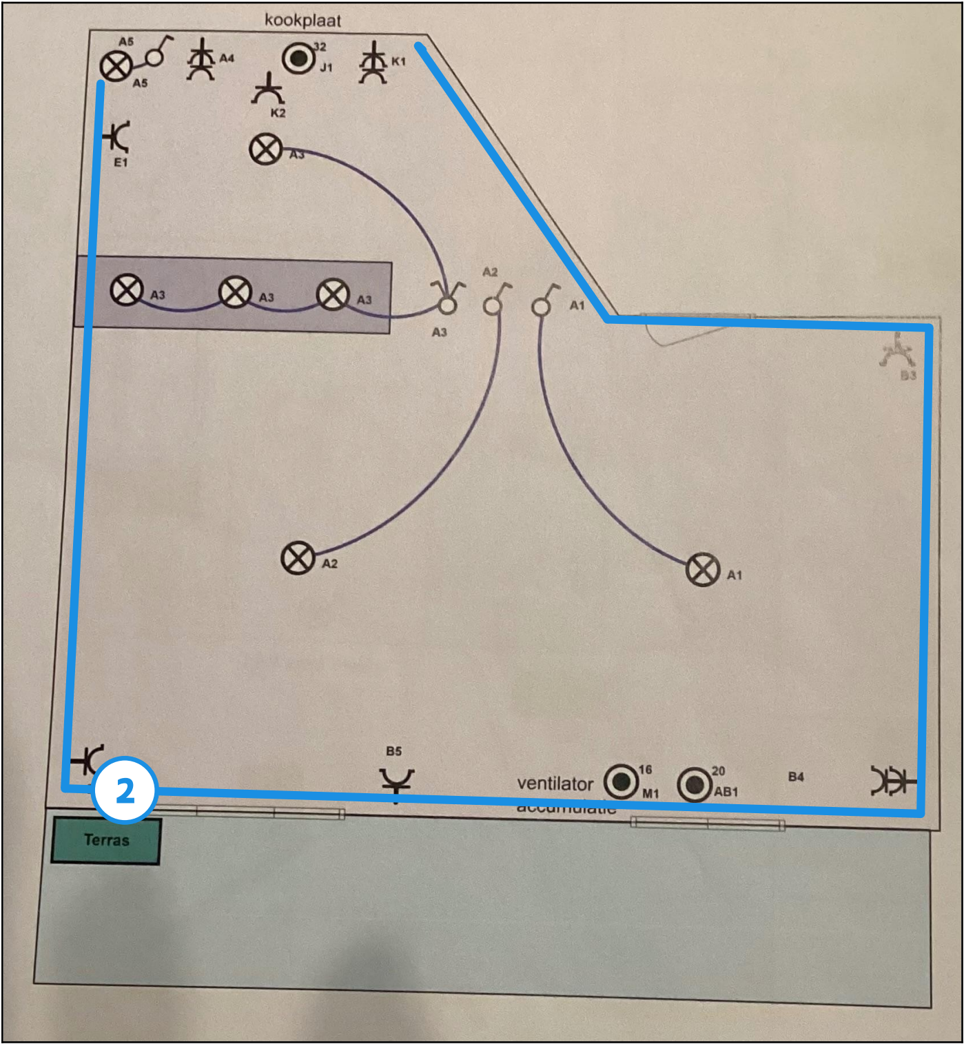
Legende van plan 1.2: Appartement 0102
