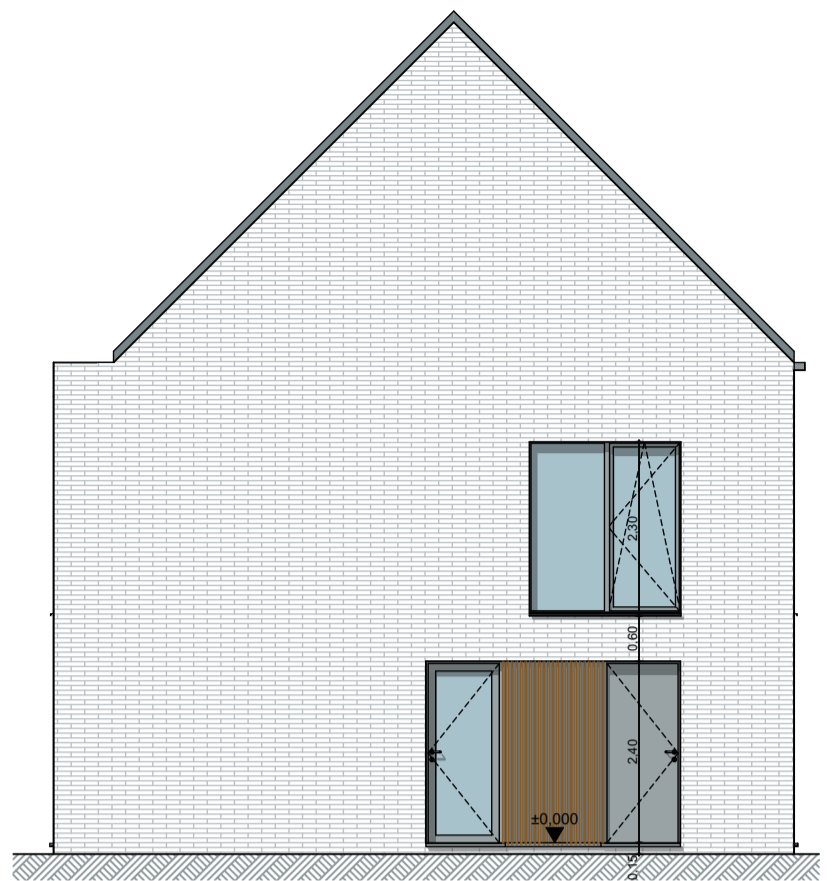
WONING 10: zijgevel links 1:100
