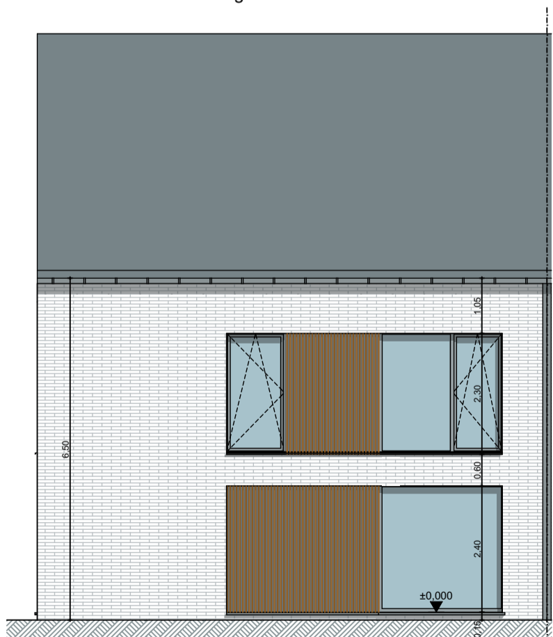
WONING 10: voorgevel 1:100
