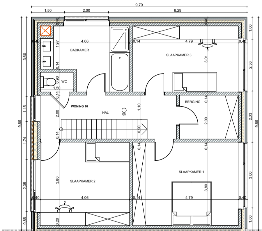
WONING 10: plan 1e verdieping 1:100
