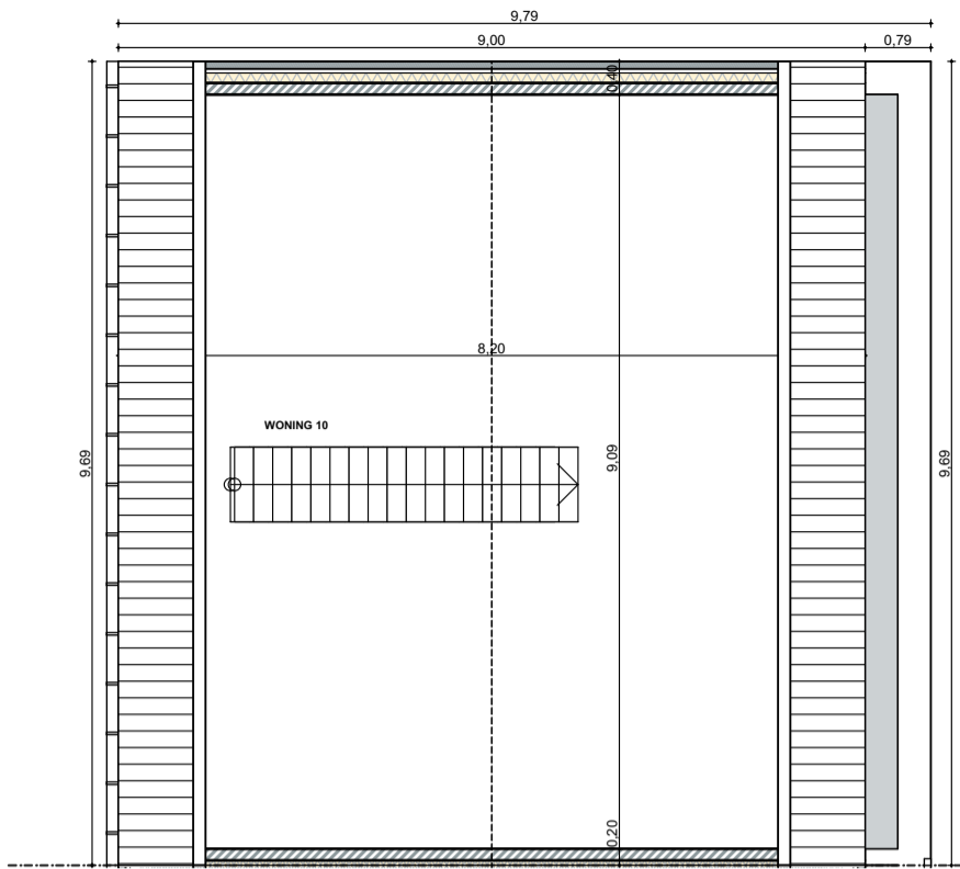
WONING 10: plan 2e verdieping 1:100
