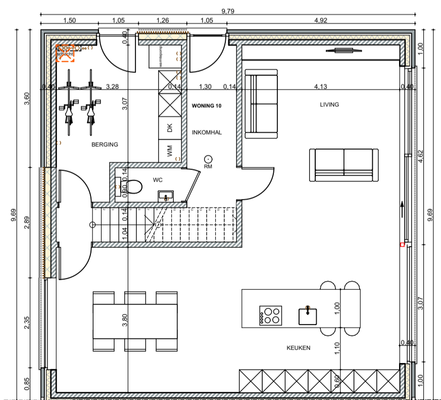
WONING 10: plan gelijkvloers 1:100
