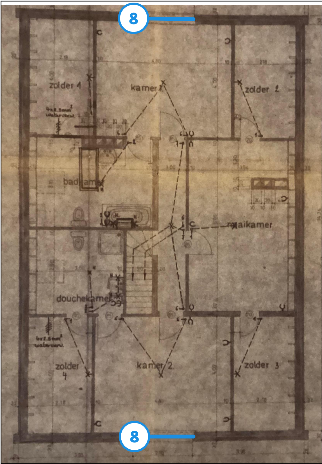
Legende van plan 1.6: Grondplan verdieping
